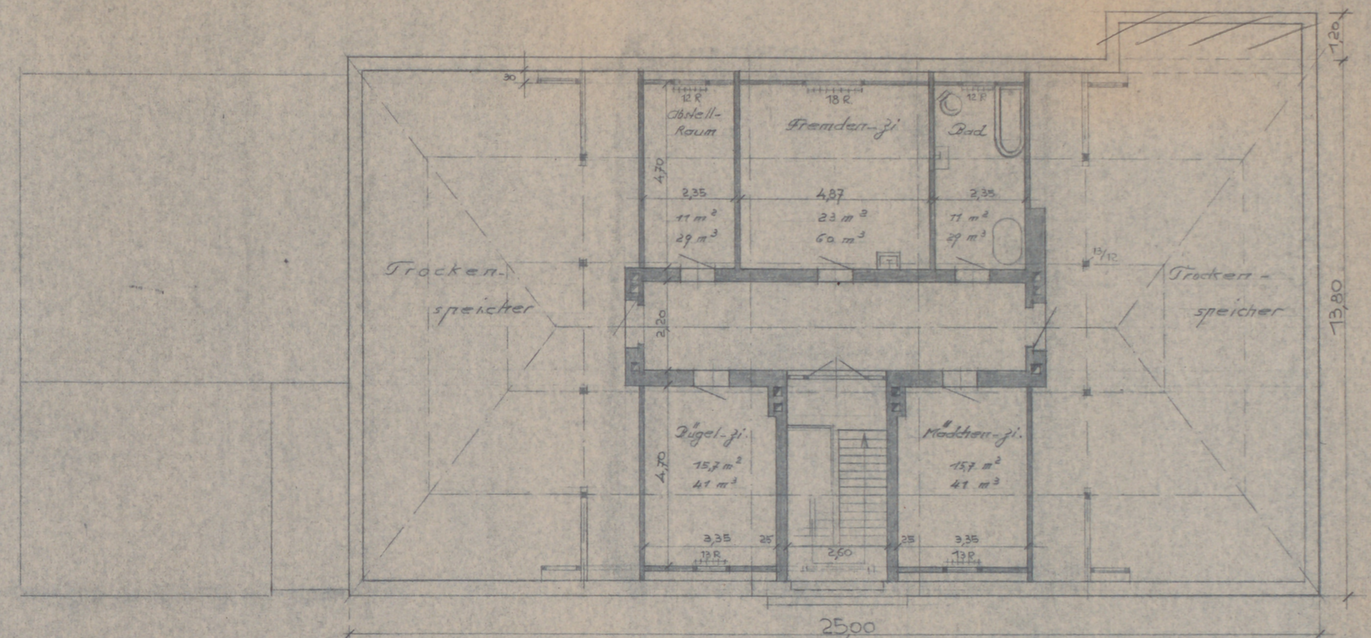
Dachgeschoß Lichte Höhe 2,90 m.
