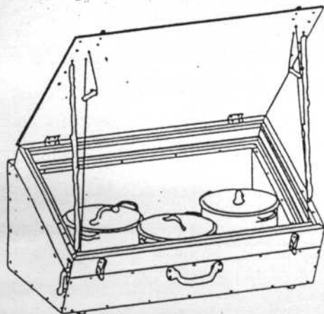
Sonnenkocher - Familienmodell für nichttropische Gebiete
