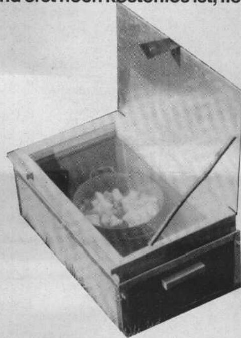
Solar-Kocher/Backofen mit einem Reflektor
