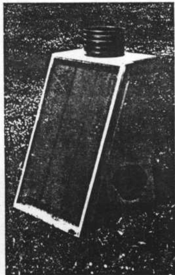
Nach dem Kaminprinzip gebaut: Sonnen-Dörrapparat
