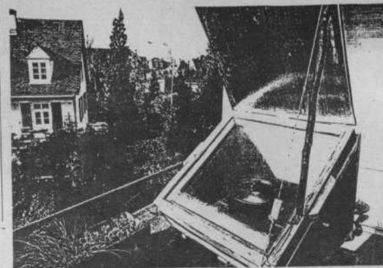
Sonnenkochkiste in Aktion: Auch im Spätherbst ist die Polenta in 2½ Stunden gar.
