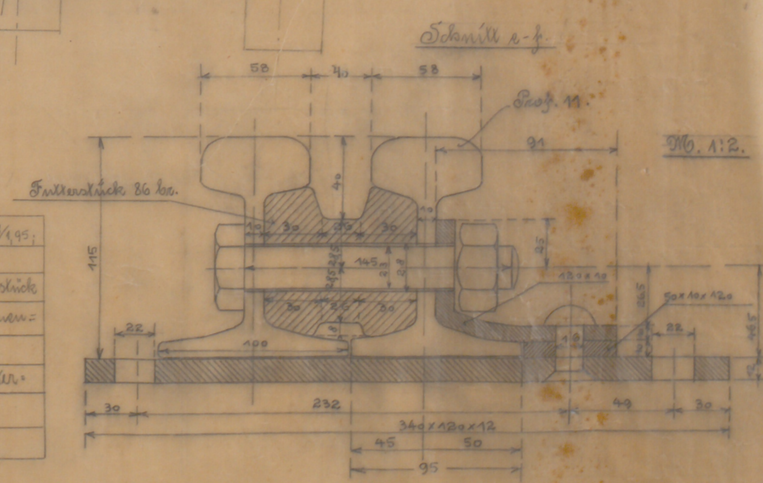
Abb. 1:10.
