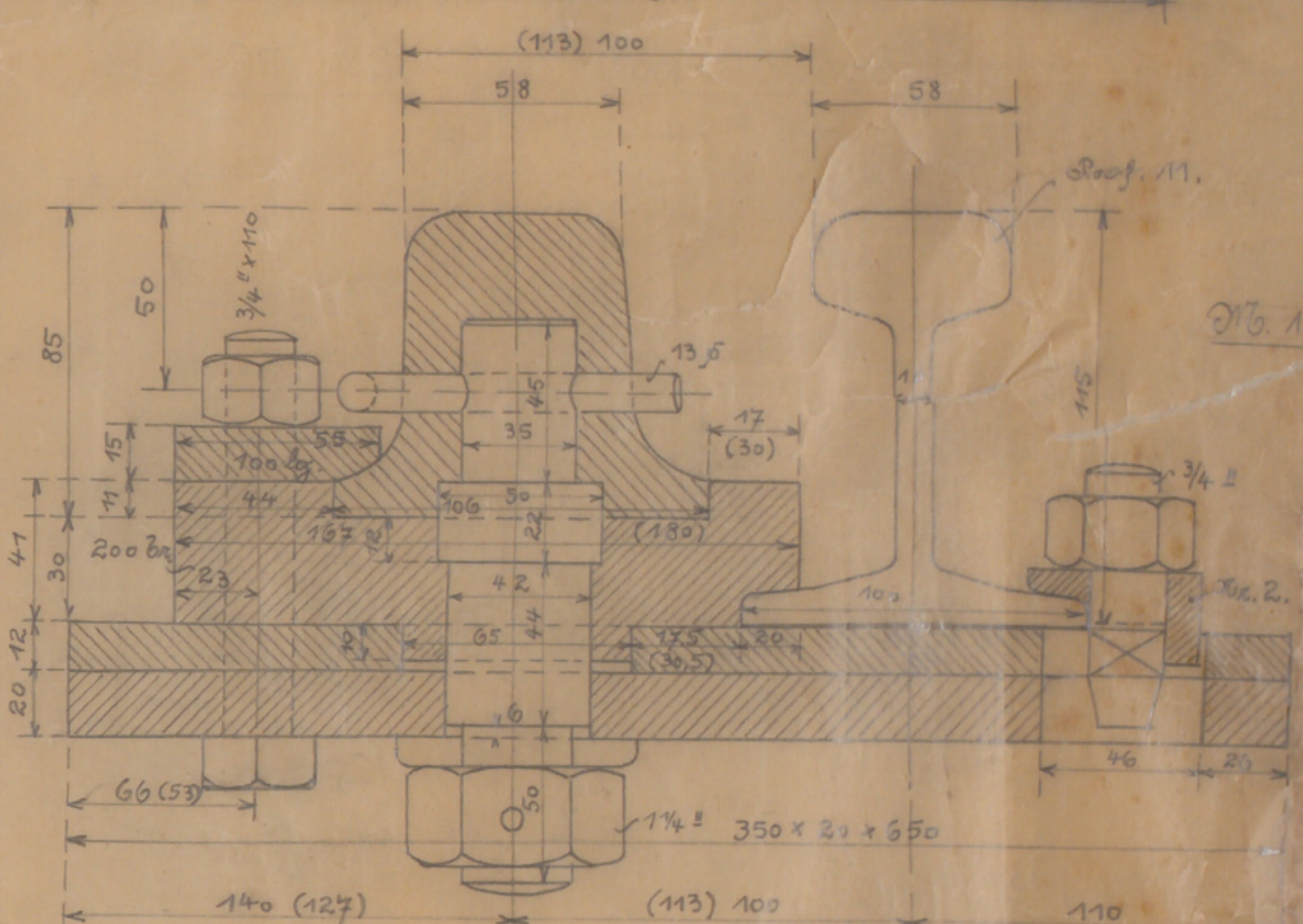
Schnitt e-f.
