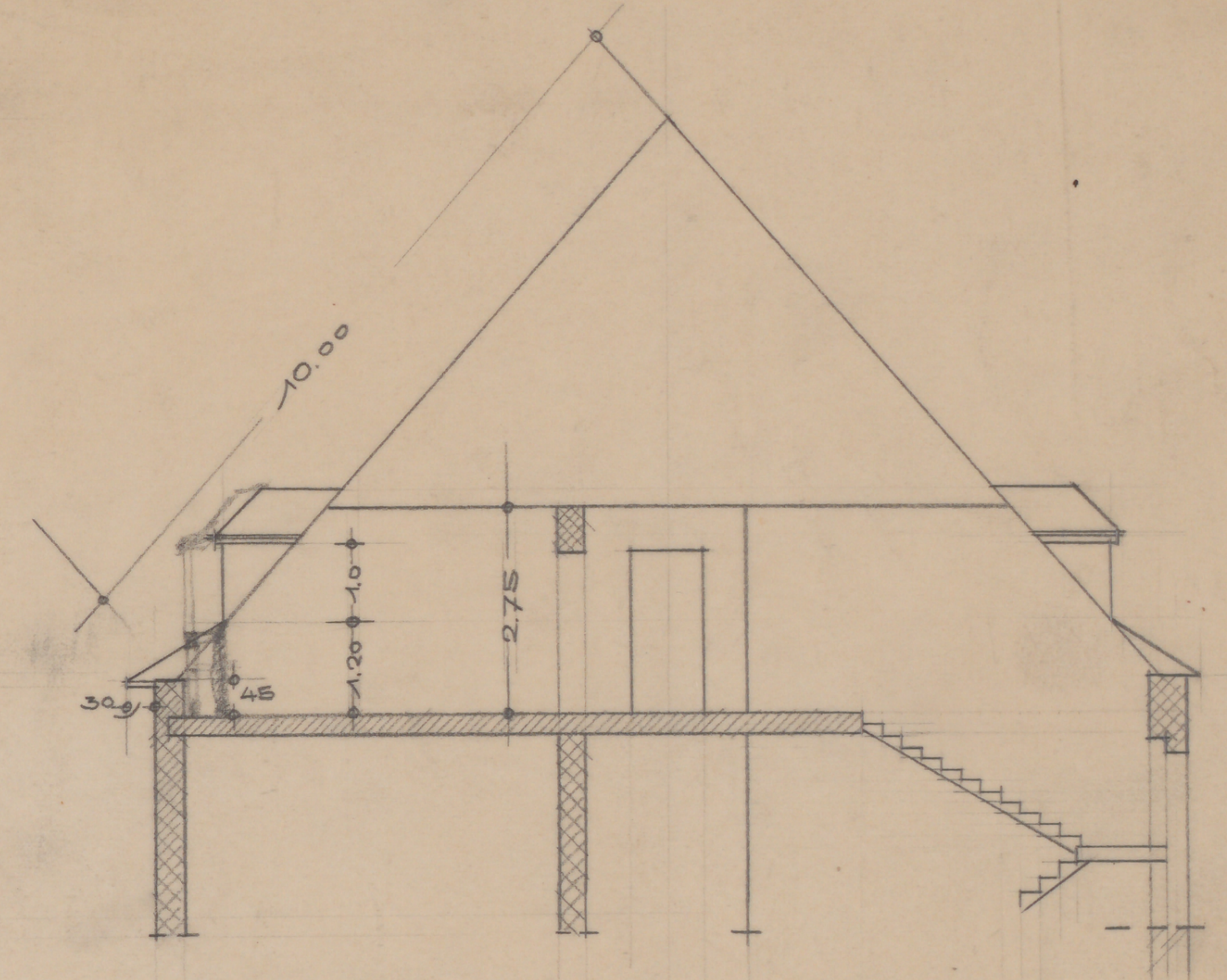
SCHNITT A-B.
