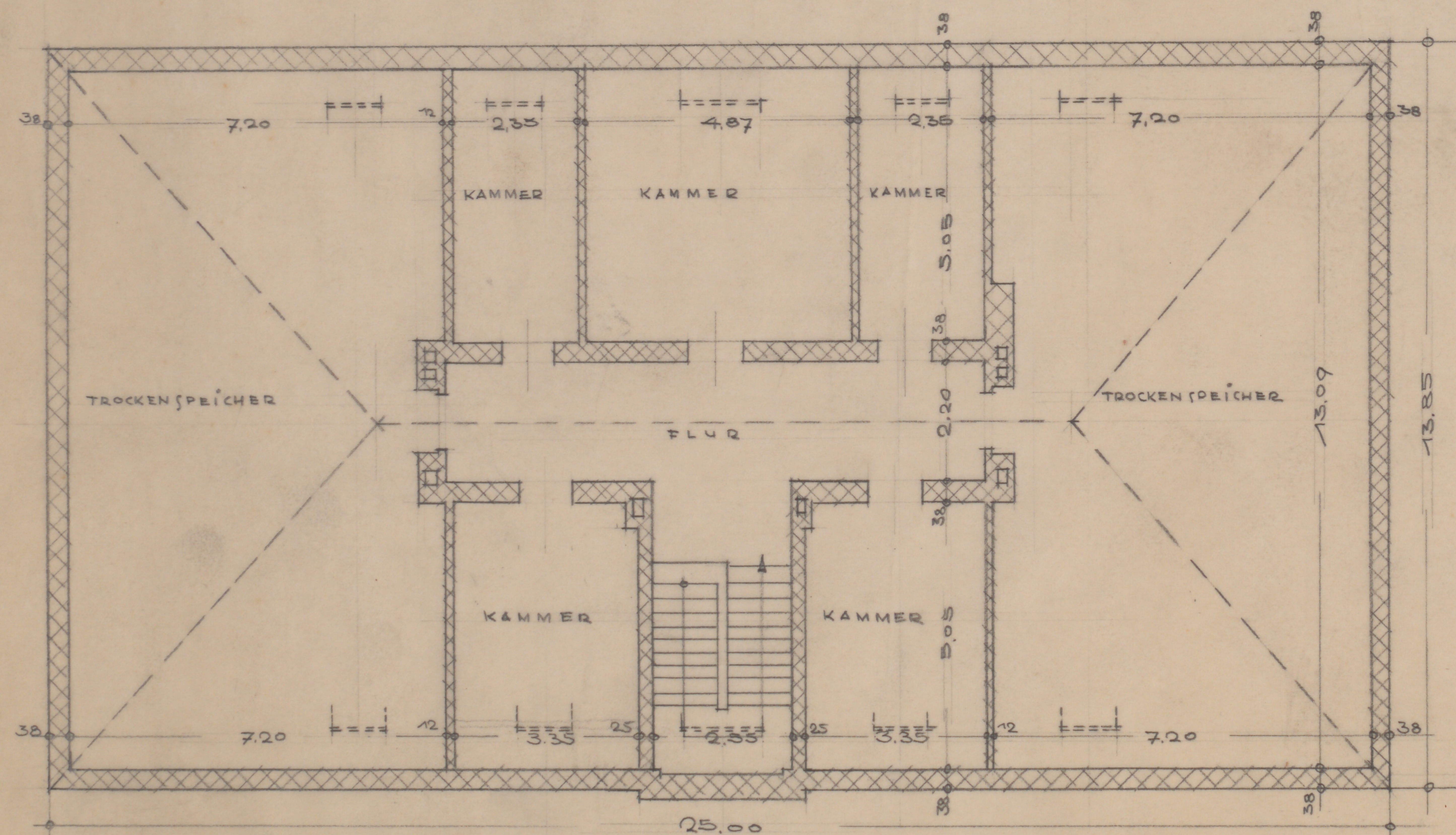
DERZEITIGER DACHGESCHOSS-GRUNDRISS.
