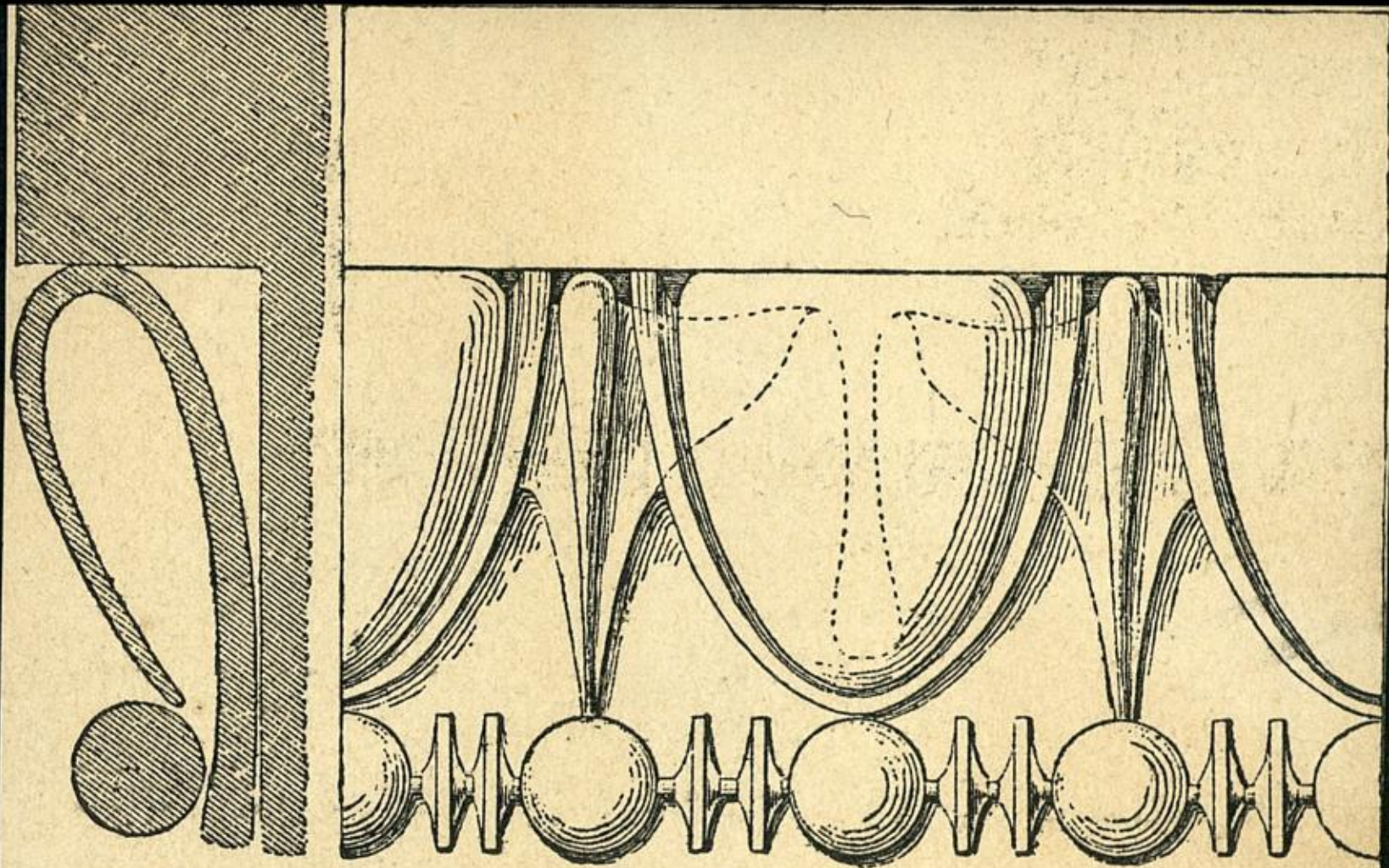
Fig. 16. Ionisches Kymation.
