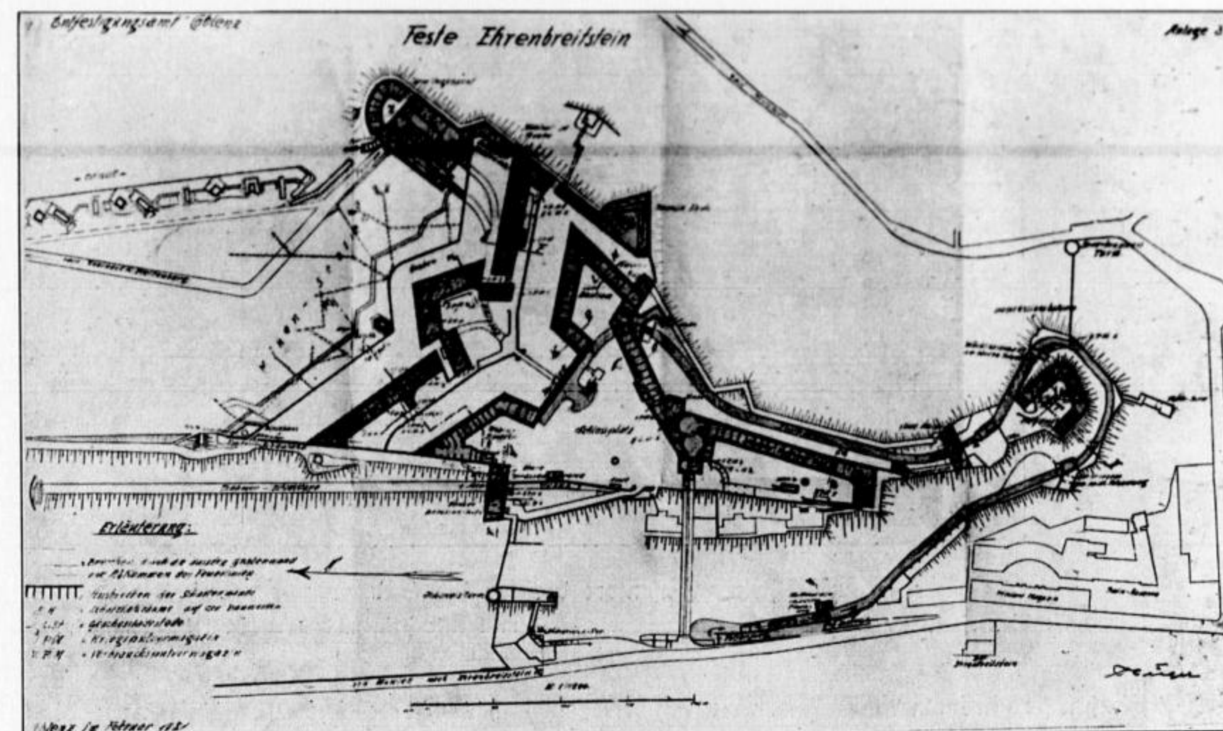
Lageplan des Ehrenbreitsteins, in der Mitte der Schloßplatz, rechts (Süden) die Südspitze und der Helfenstein.
