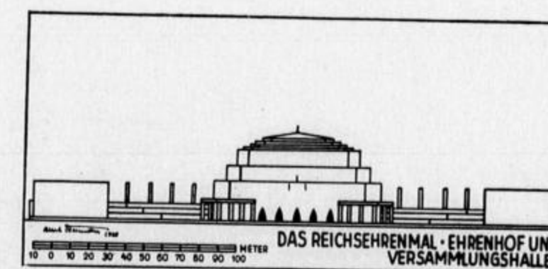
Ehrenhof mit Versammlungsraum. Schmalseite.
