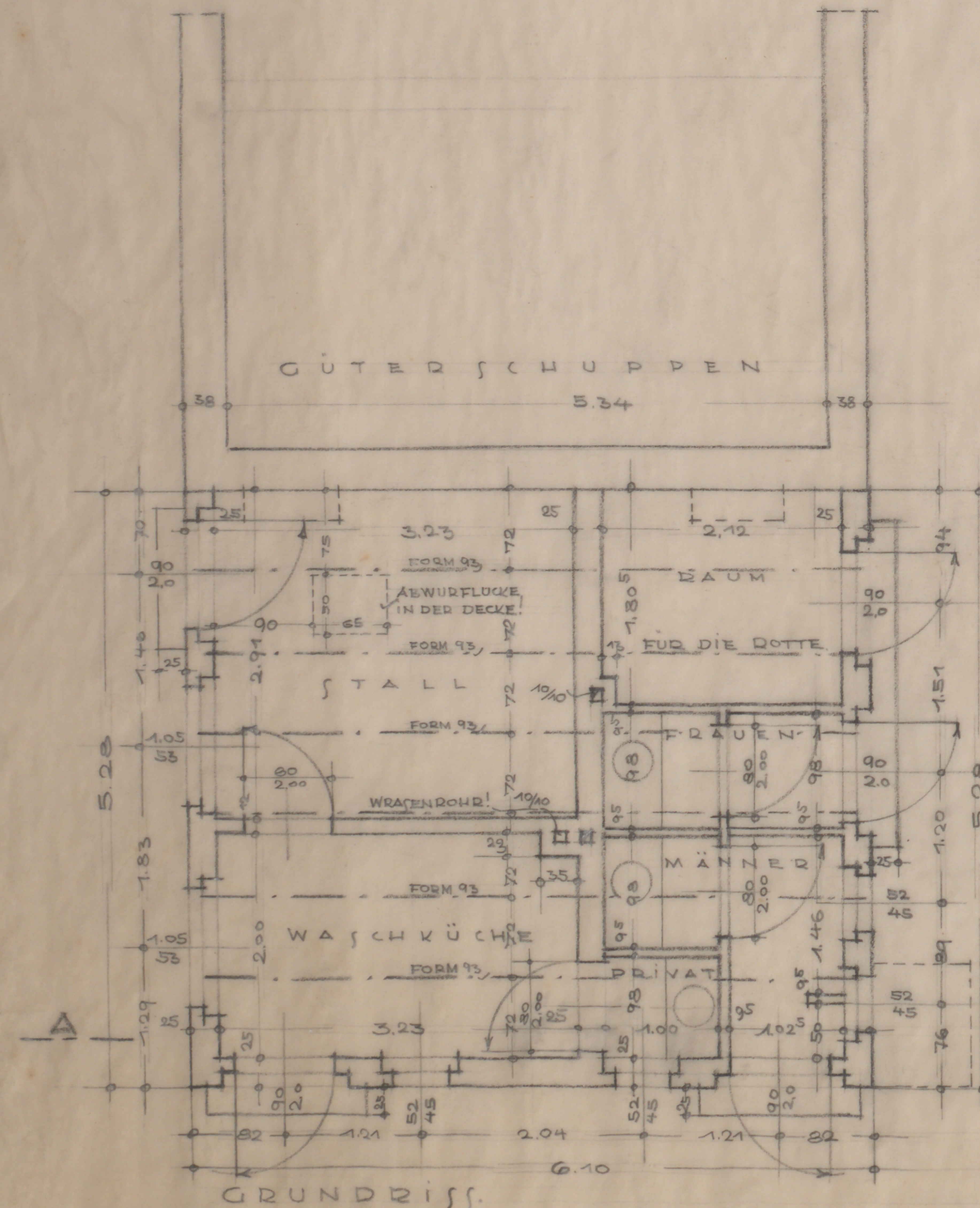
GRUNDRISS.
