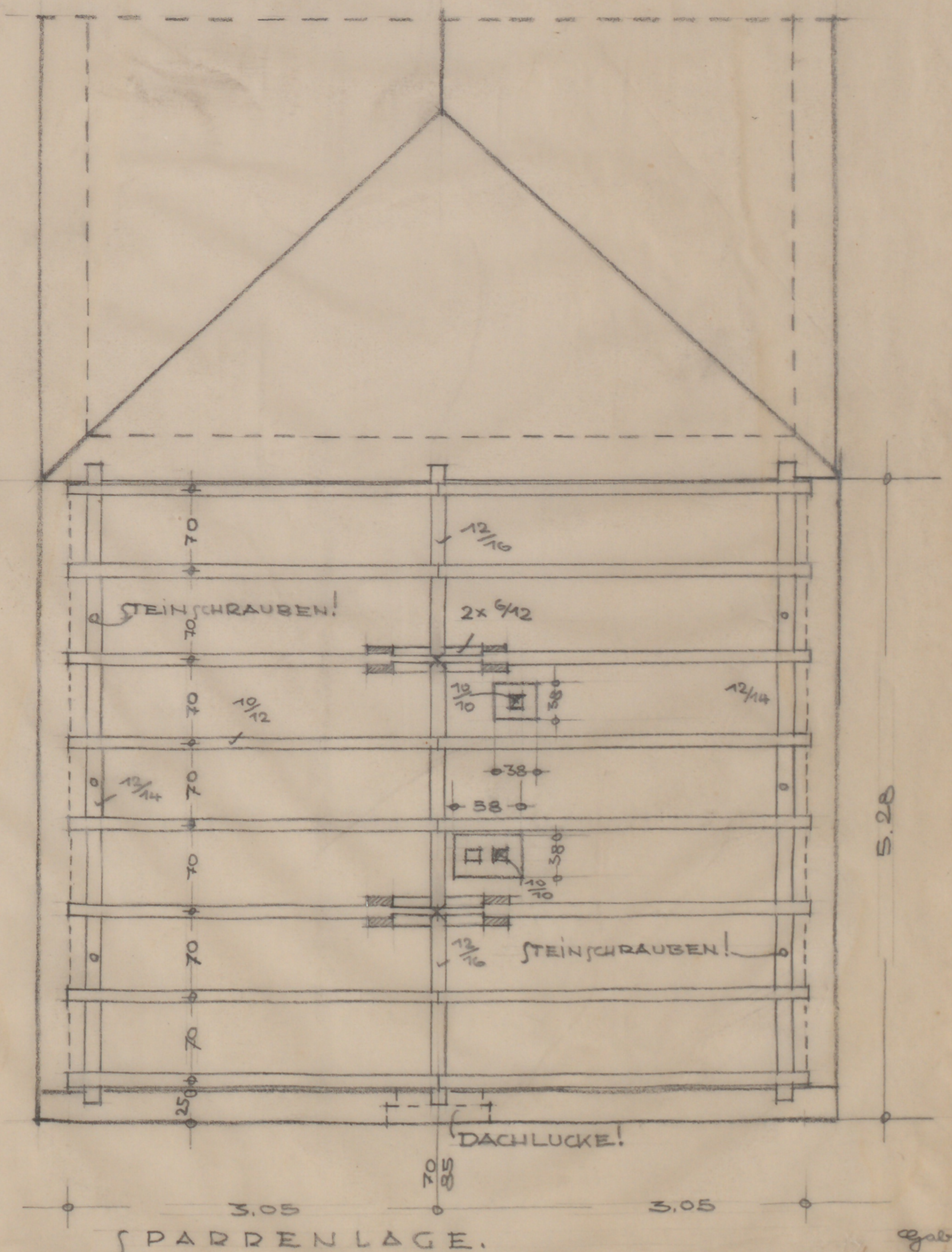
DACHSTUHL.
