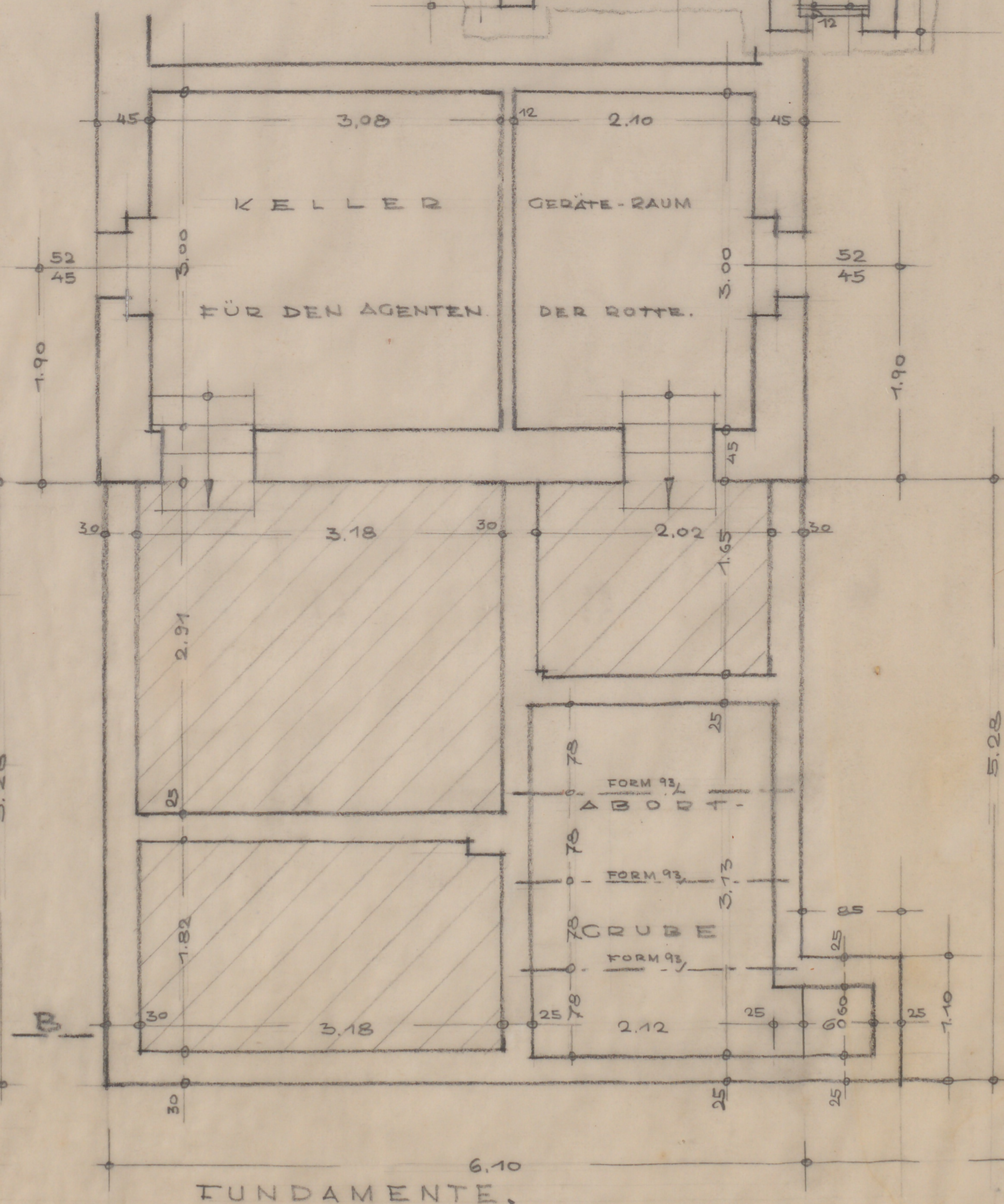
FUNDAMENTE.
