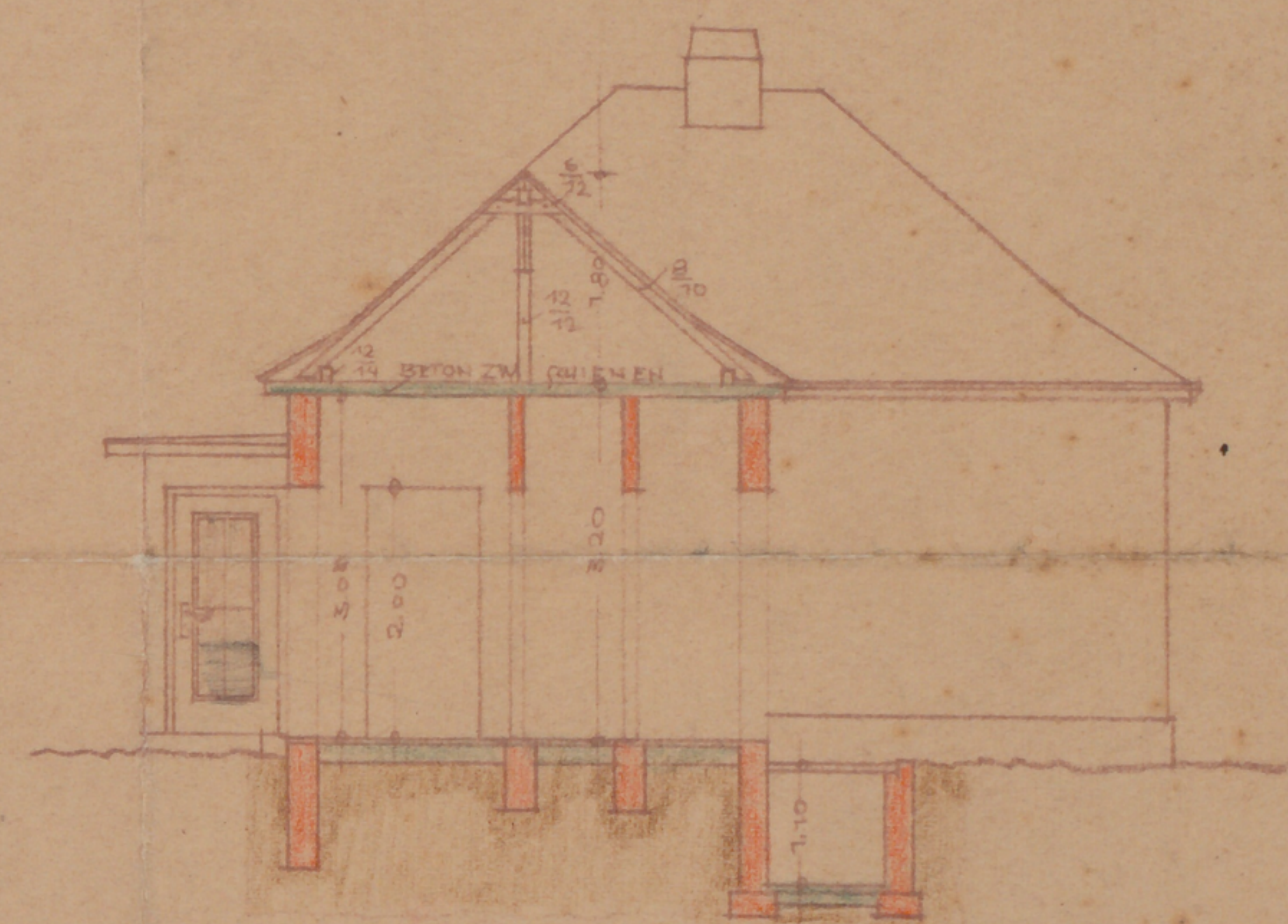
SNITT A-B.
