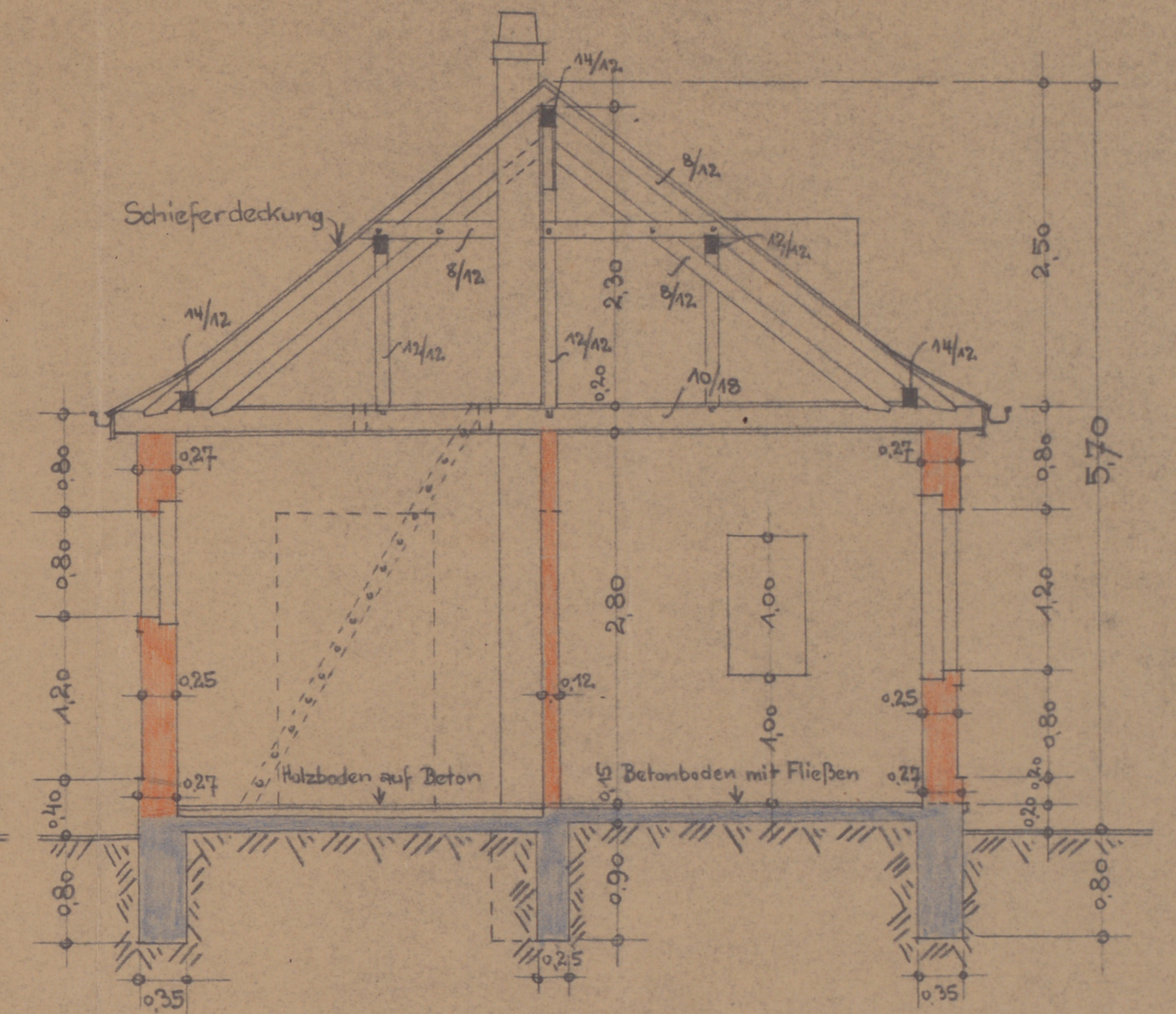
Schnitt a-b.
