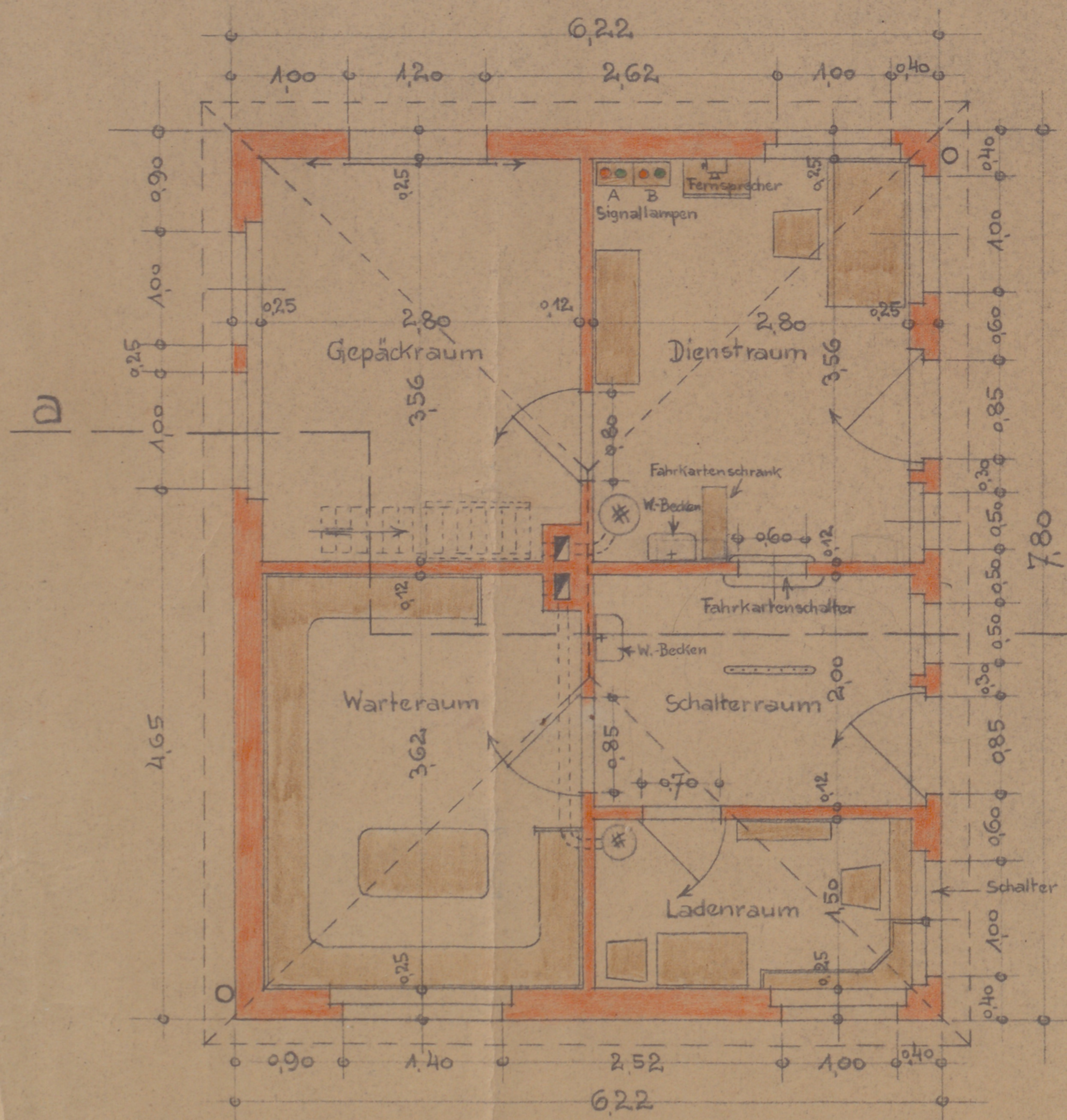
Grundriß.
