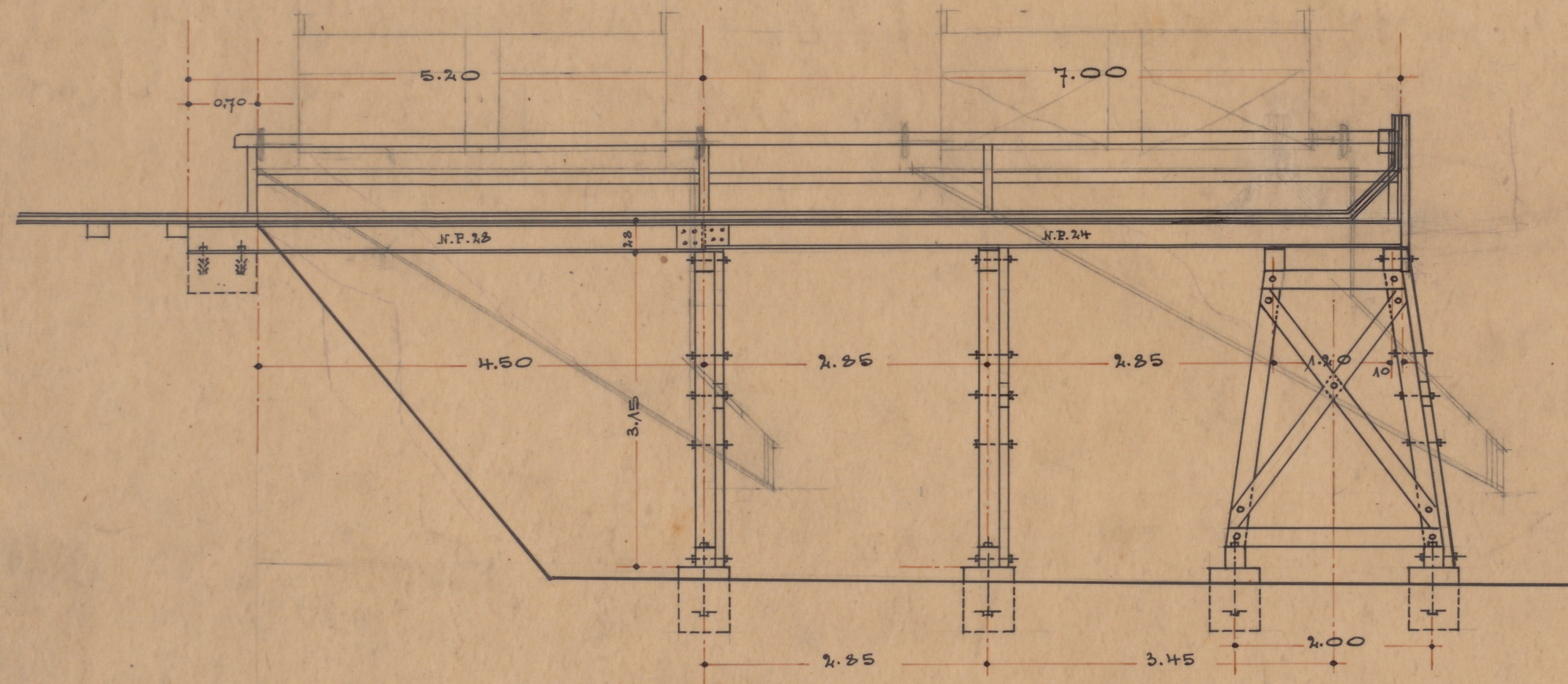
Längenschnitt.
