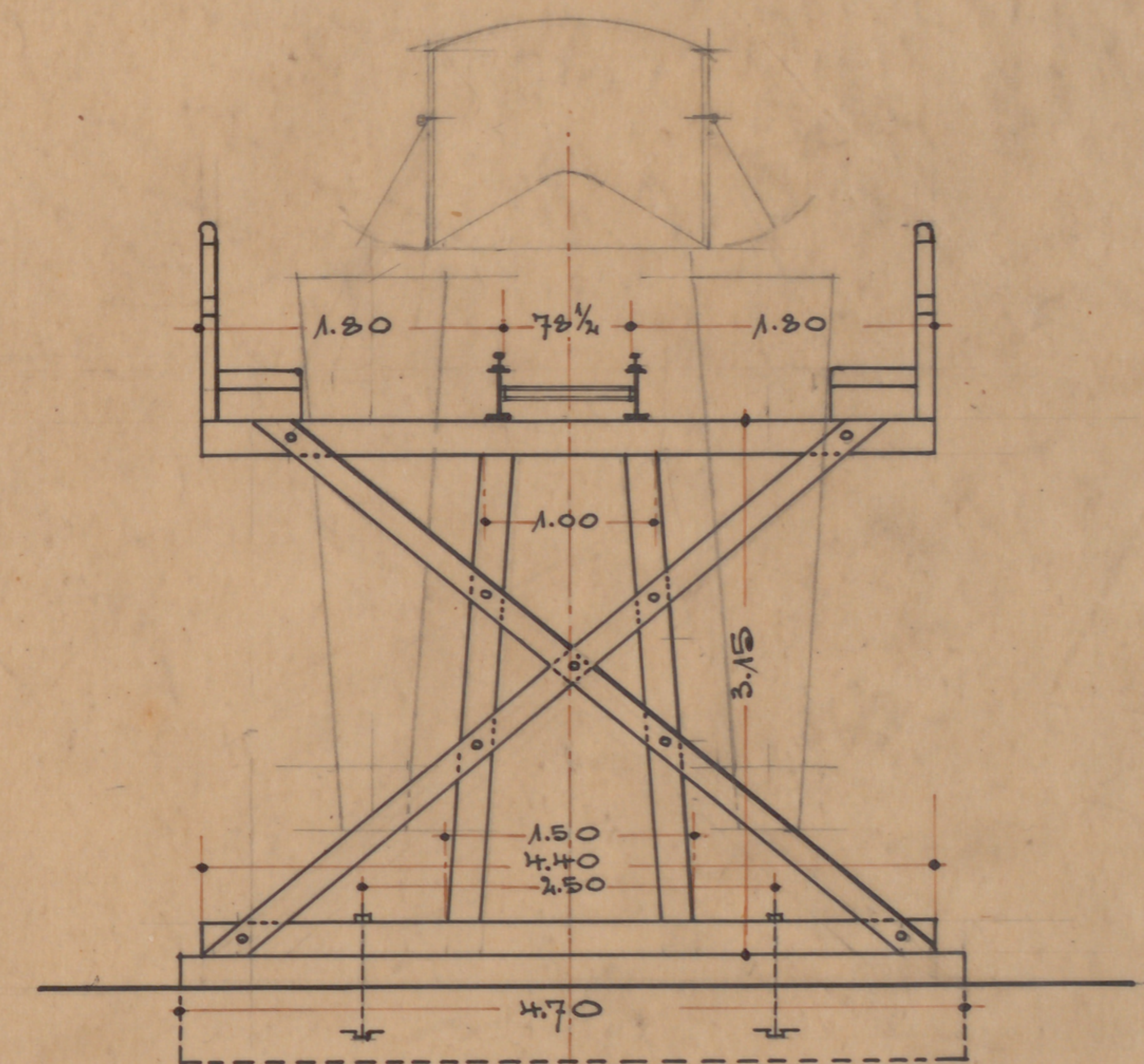
Querschnitt.
