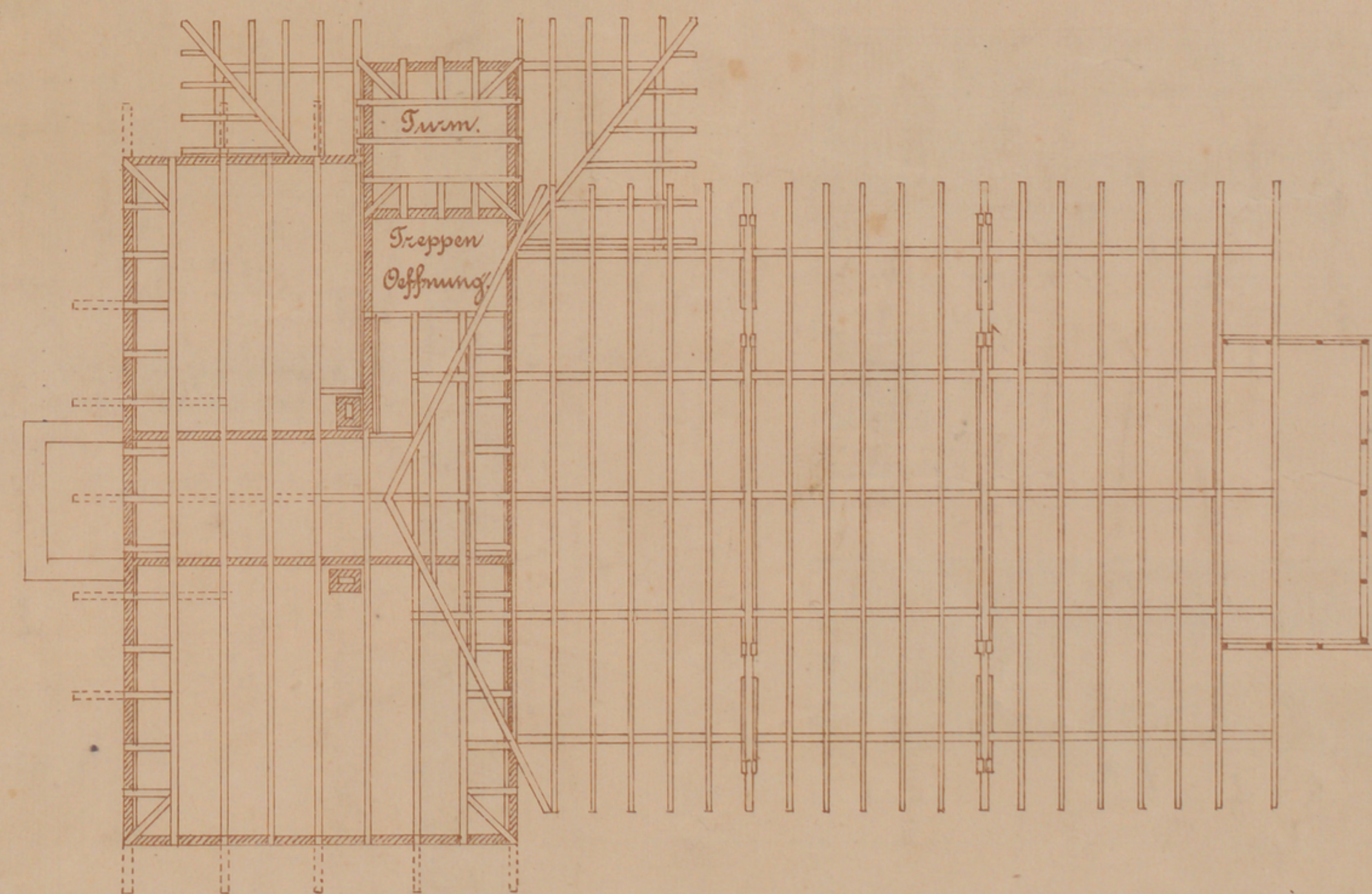
Zweite Balkenlage nebst Pfetten- und Sparrenlage.
