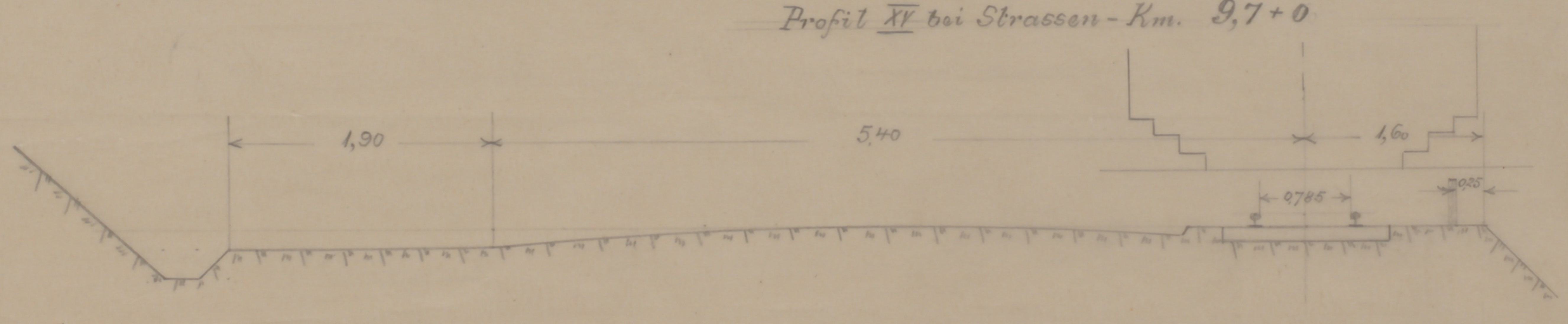
Profil XVI bei Strassen-Km. 11,8+50
