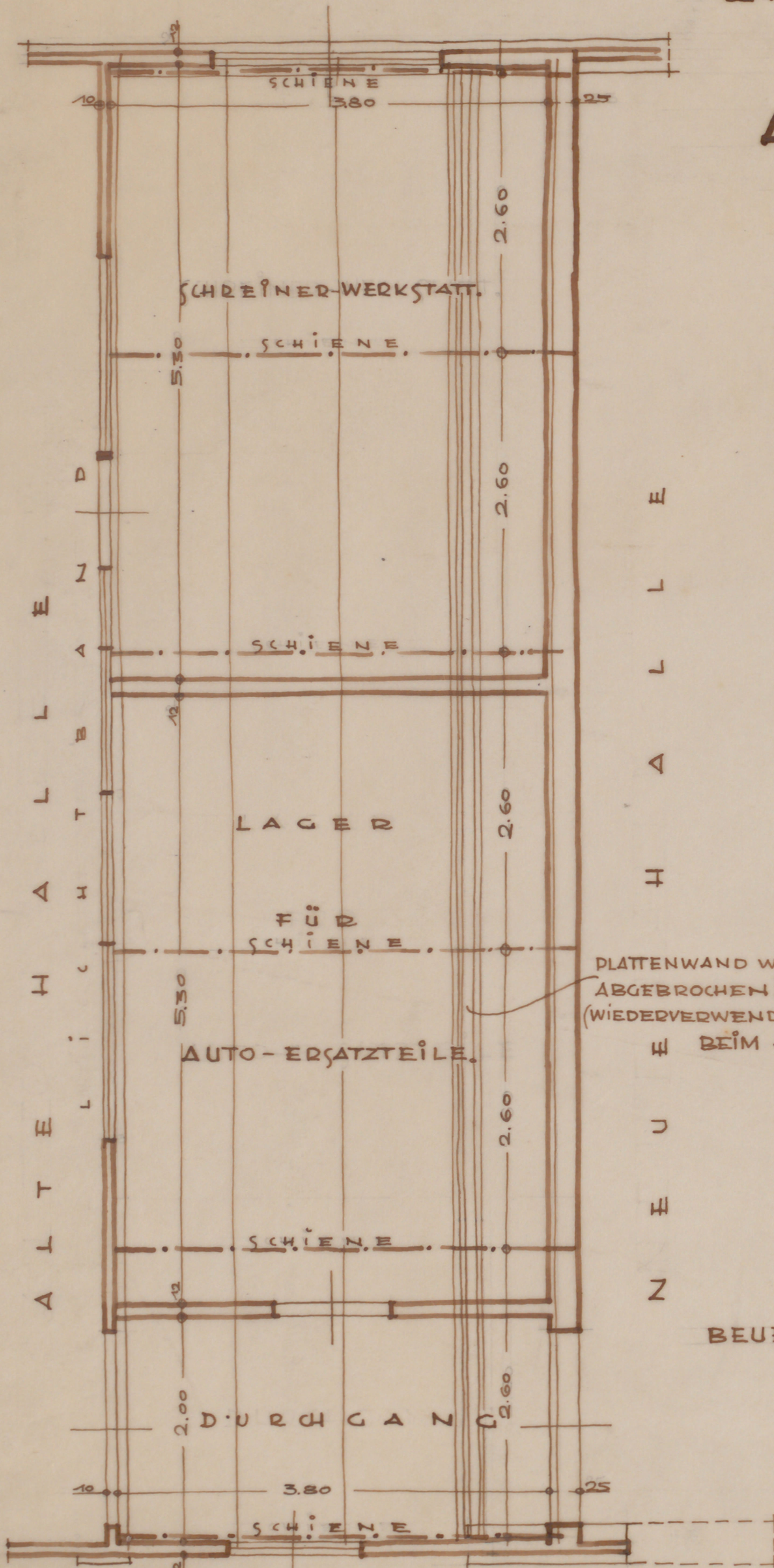
GRUNDRISS. (ZWISCHENBAU).
