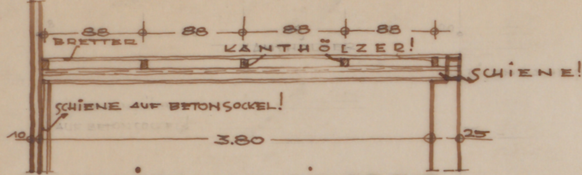
SNITT DURCH DIE DECKE.
