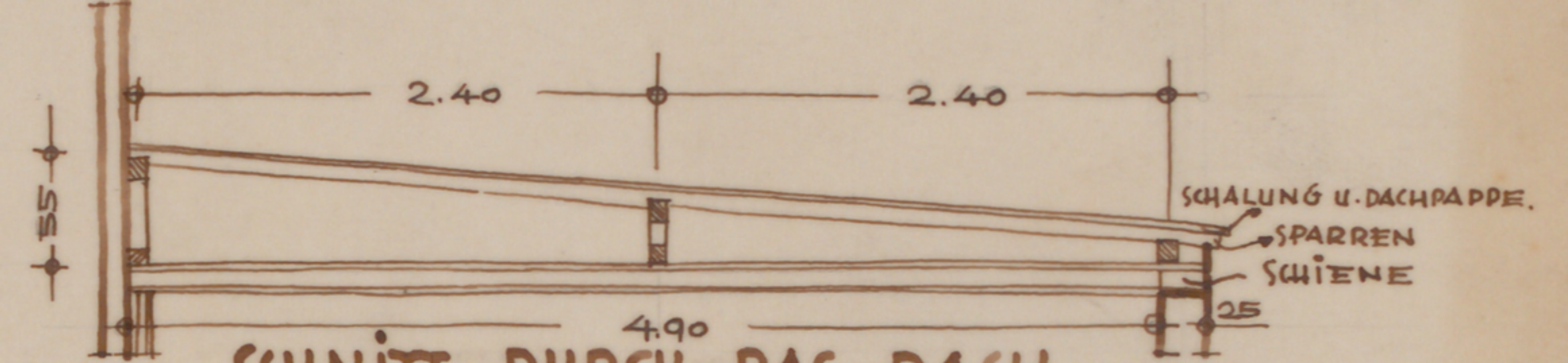
SNITT DURCH DAS DACH.
