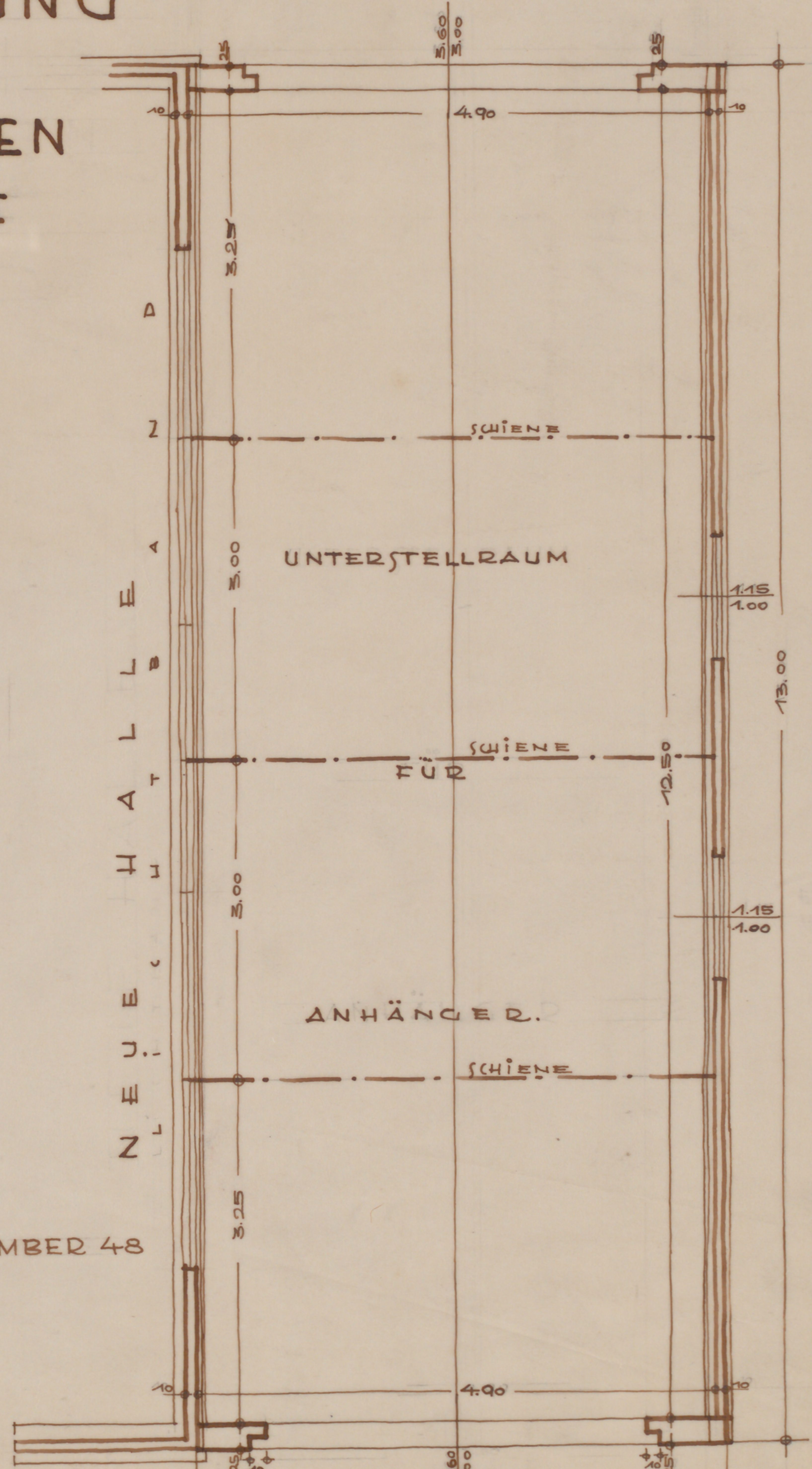
GRUNDRISS. (ANBAU).
