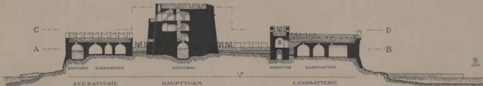
LÄNGSCHNITT E-F
