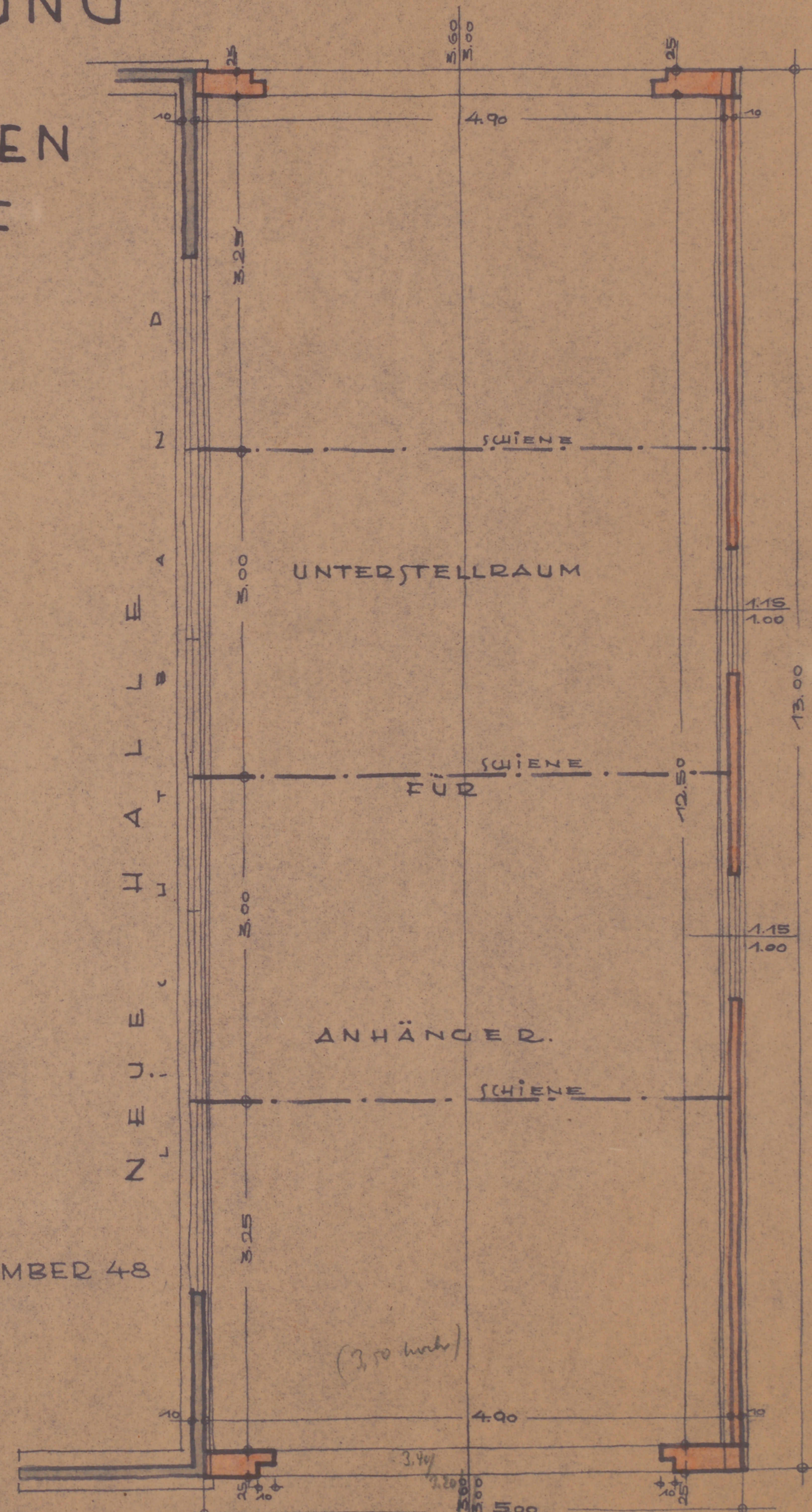
GRUNDRISS (ANBAU).
