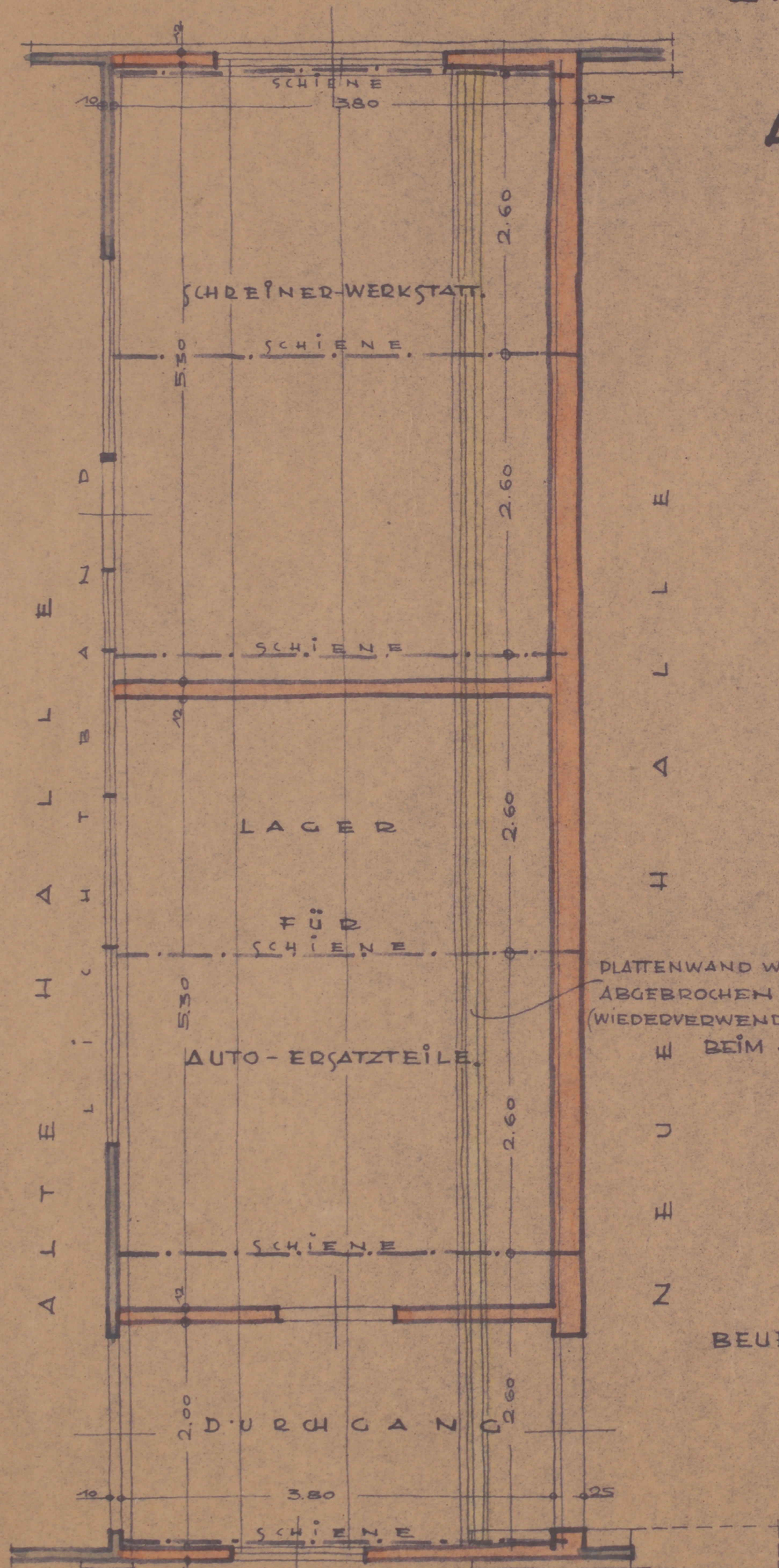
GRUNDRISS (ZWISCHENBAU).
