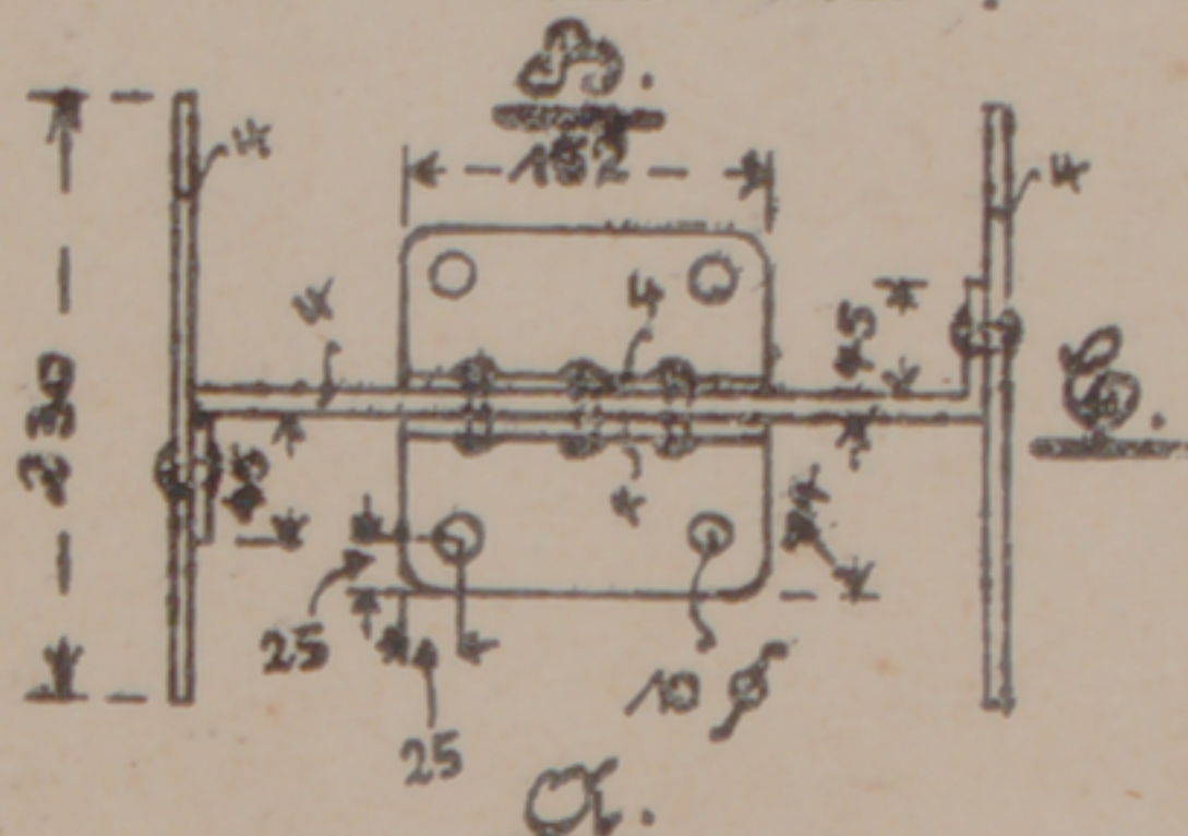
Seitenansicht.
