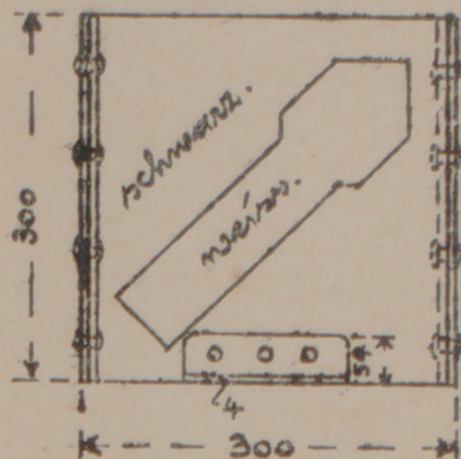
Ansicht A.
