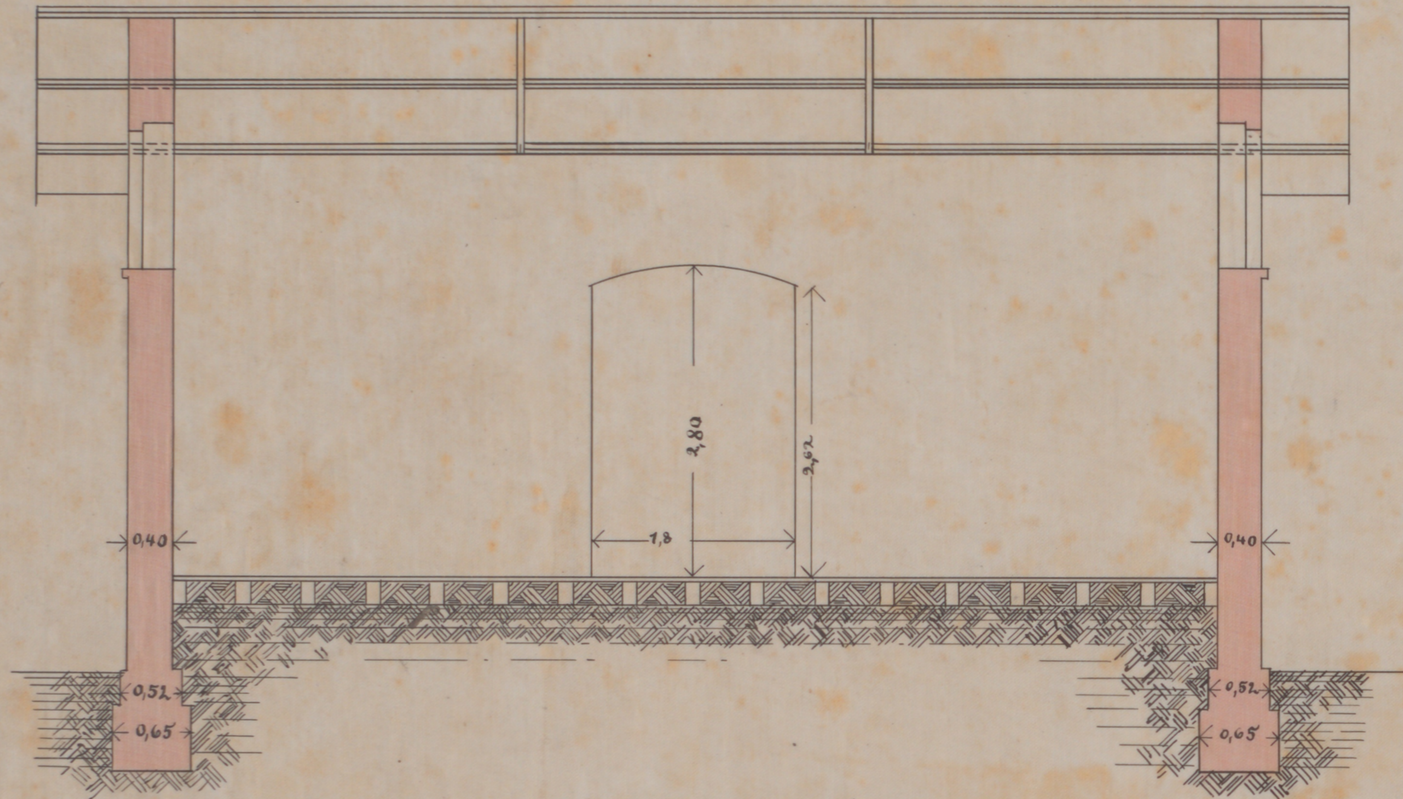
Längenschnitt.
