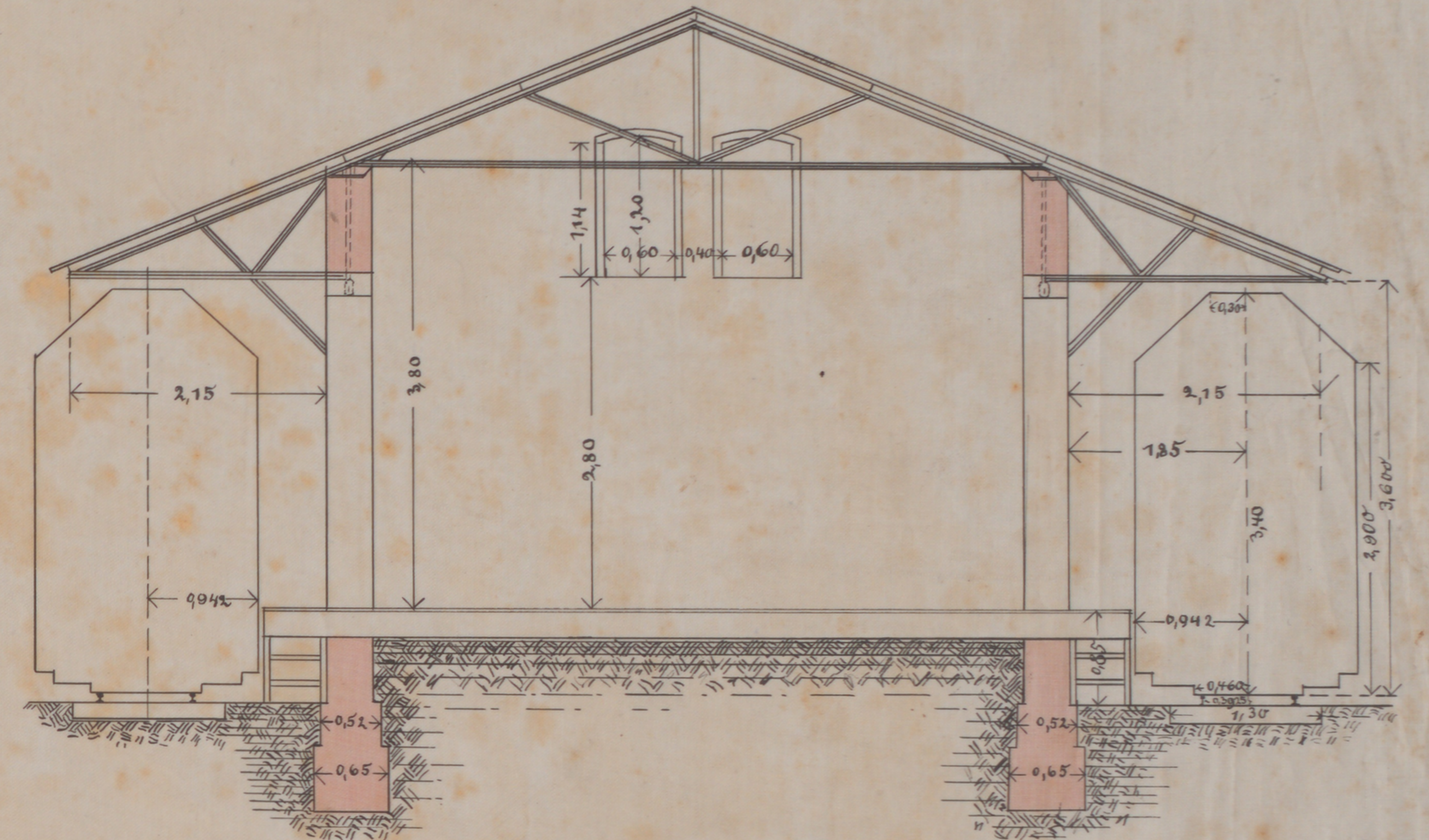
Querschnitt.
