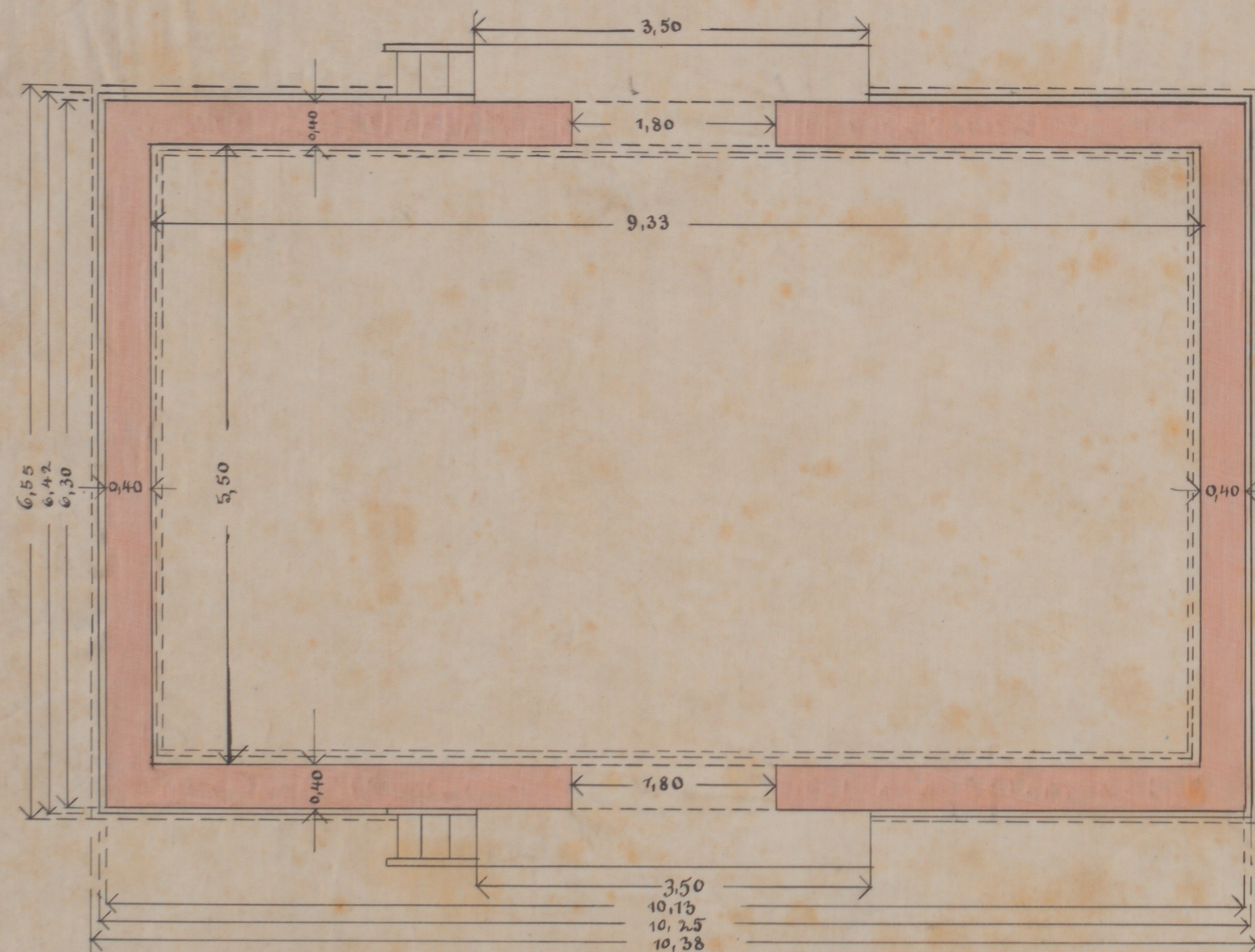
Grundriss.
