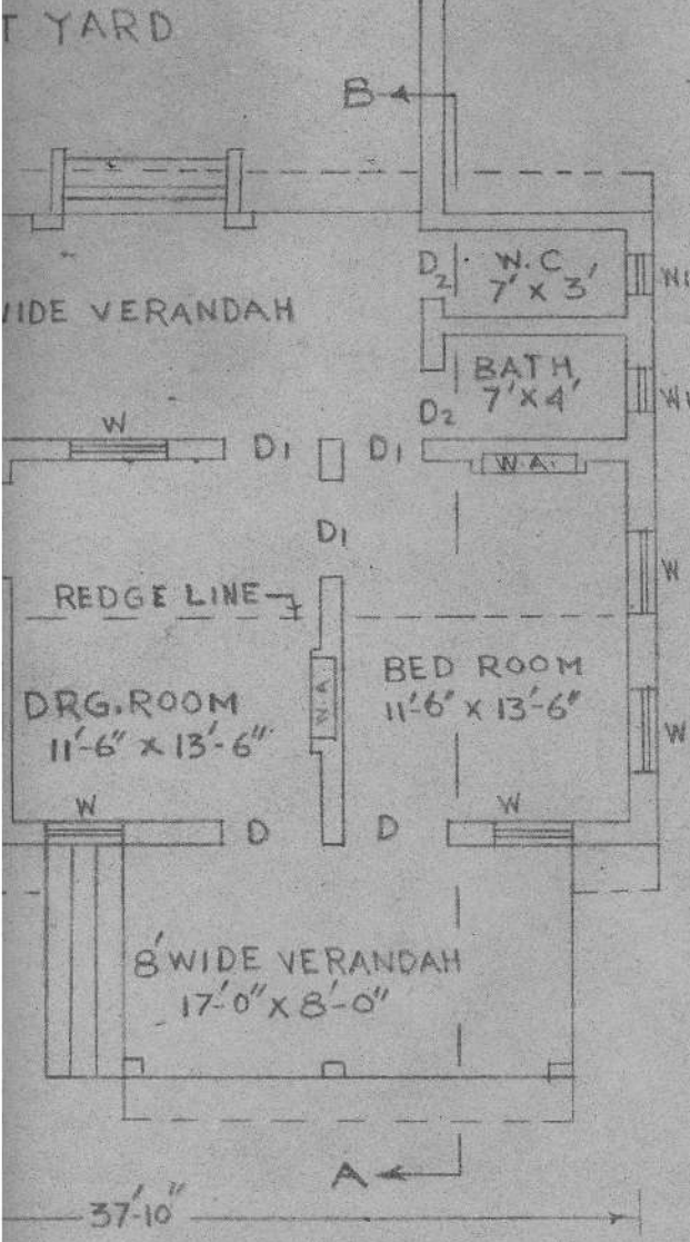
PLAN SCALE: 1"=8'
