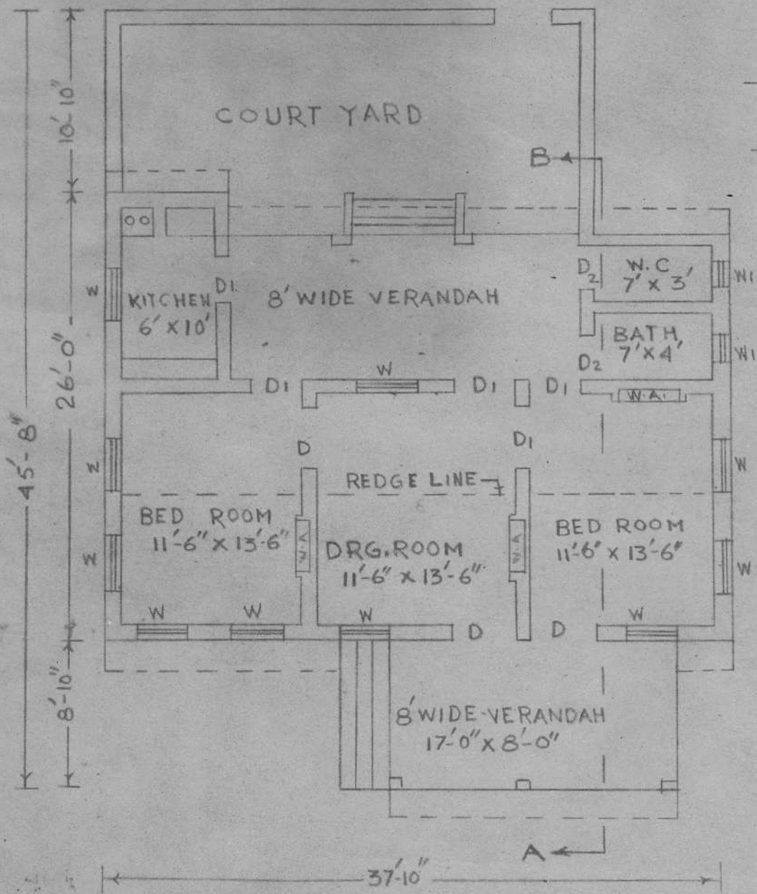
PLAN SCALE: 1" = 8'
