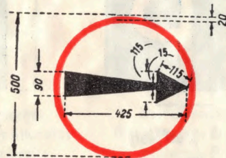
Rechts bzw. Links Nr. 24
