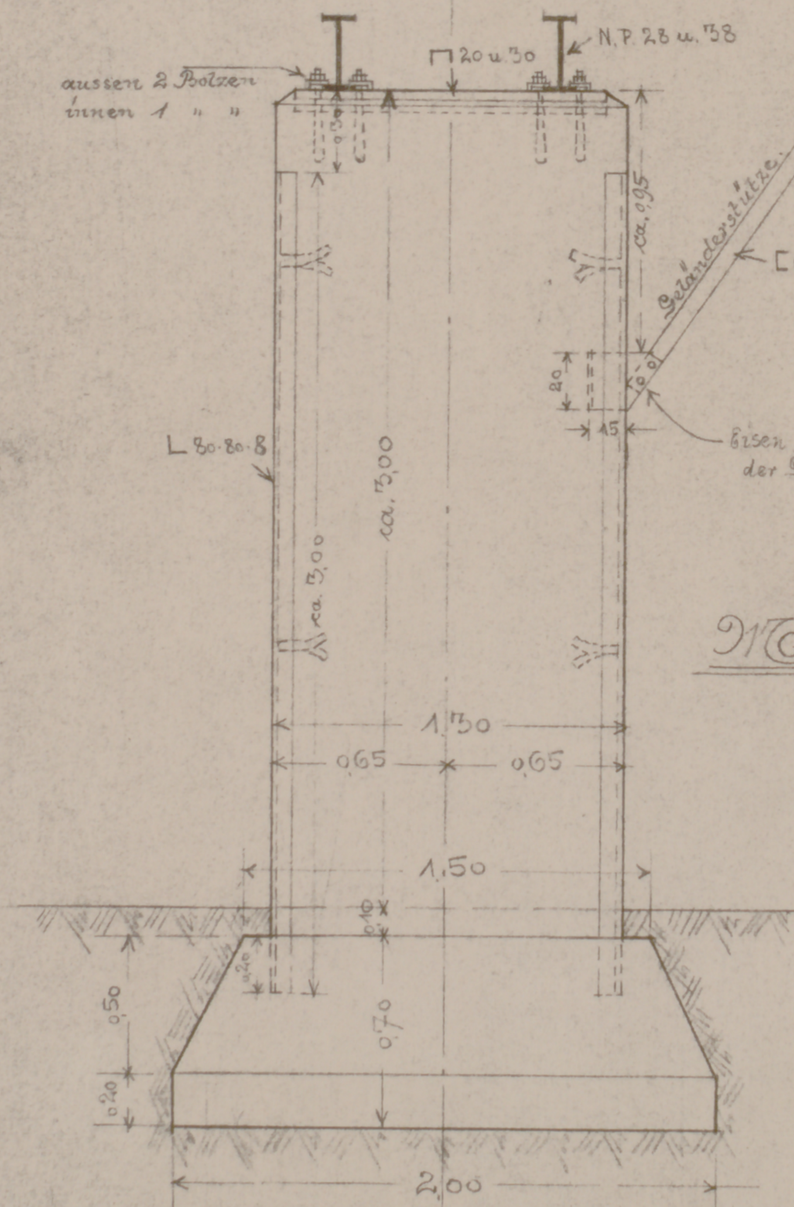
Seitenansicht. (Längsrichtung)
