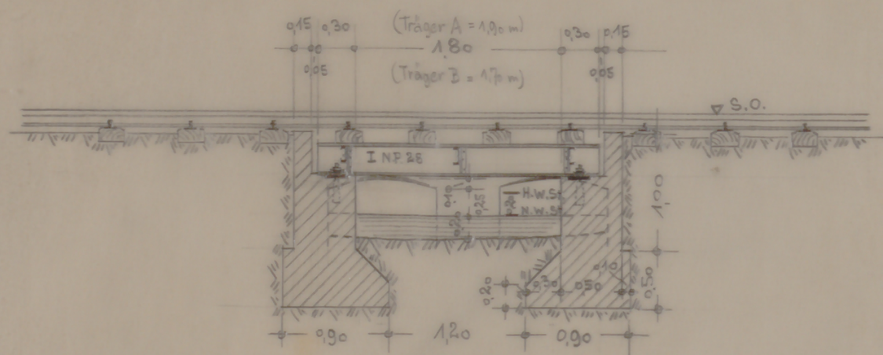
Längenschnitt a-b.
