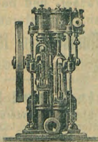
Klein's Compoundpumpe mit nur einem Schieber.
