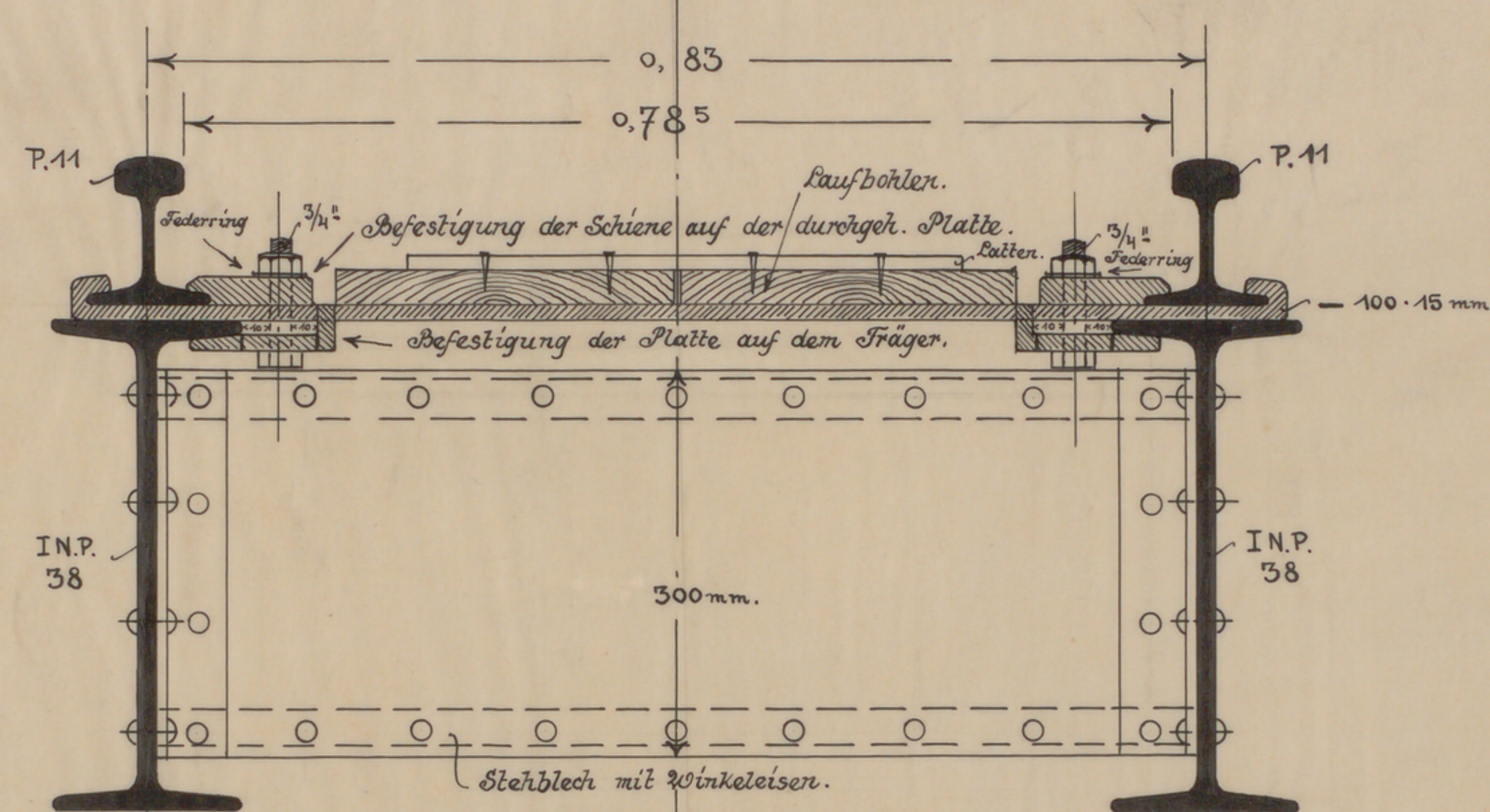
Schnitt N. P. 38.
