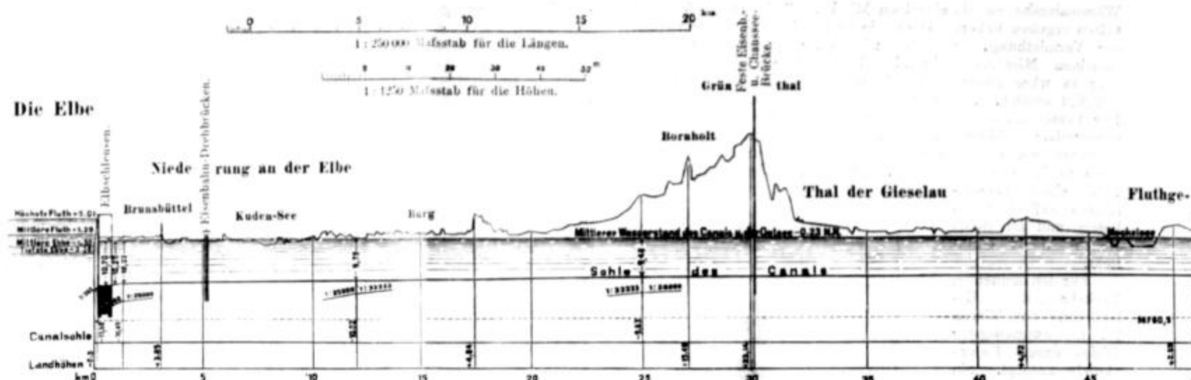
Abb. 2. Längenschnitt des
