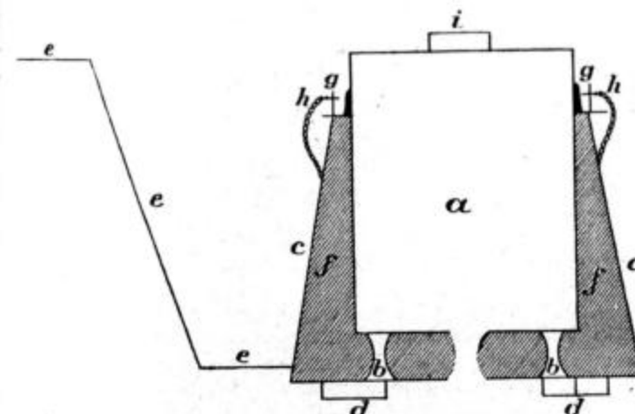
a Blechcylinder außen latirt mit Füssen b. c Holzmantel etwas niedriger wie e und nicht zu weit zu nehmen. d Untermauerung. e Dampfzuführung. f Wasser. g 3 Eisenbäden an a befestigt. h 3 durchlöchte Eisenstifte in c be- festigt. i 2 Handgriffe.
