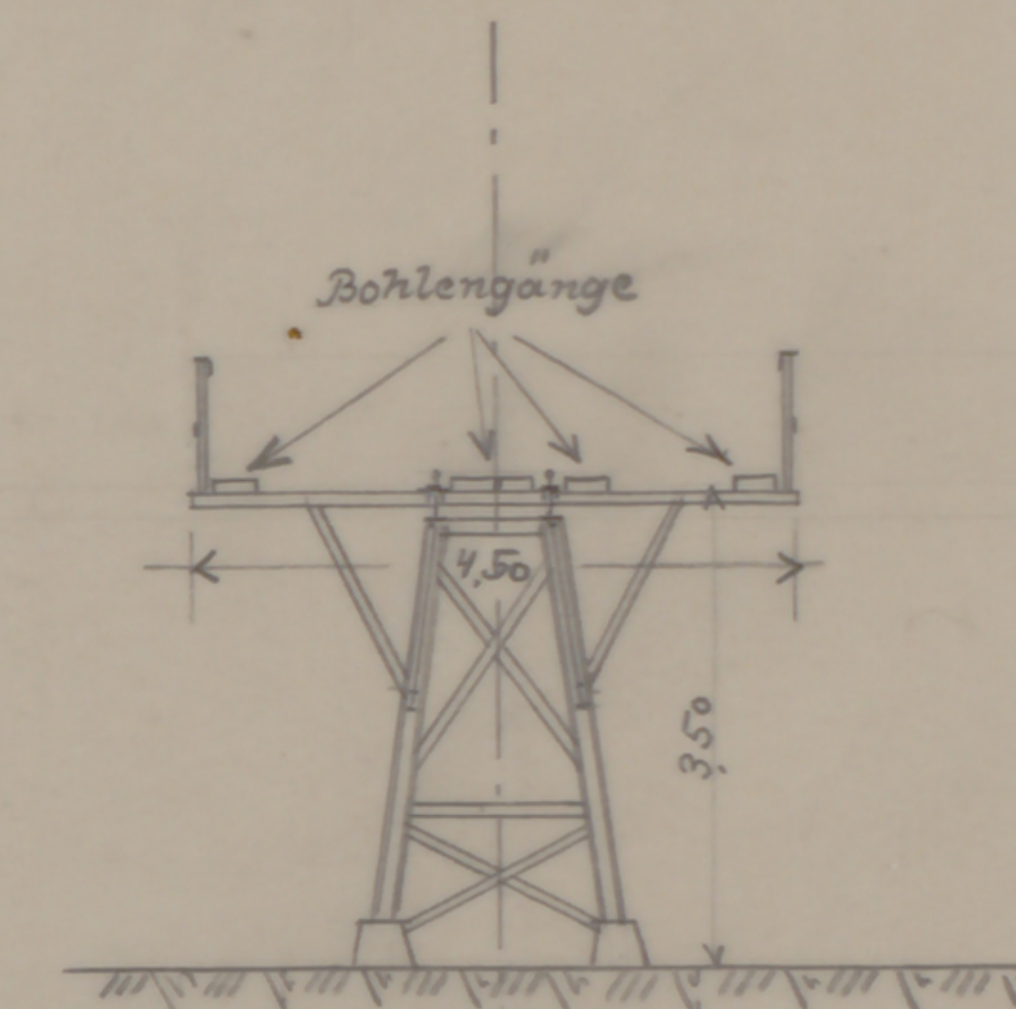
Schnitt.
