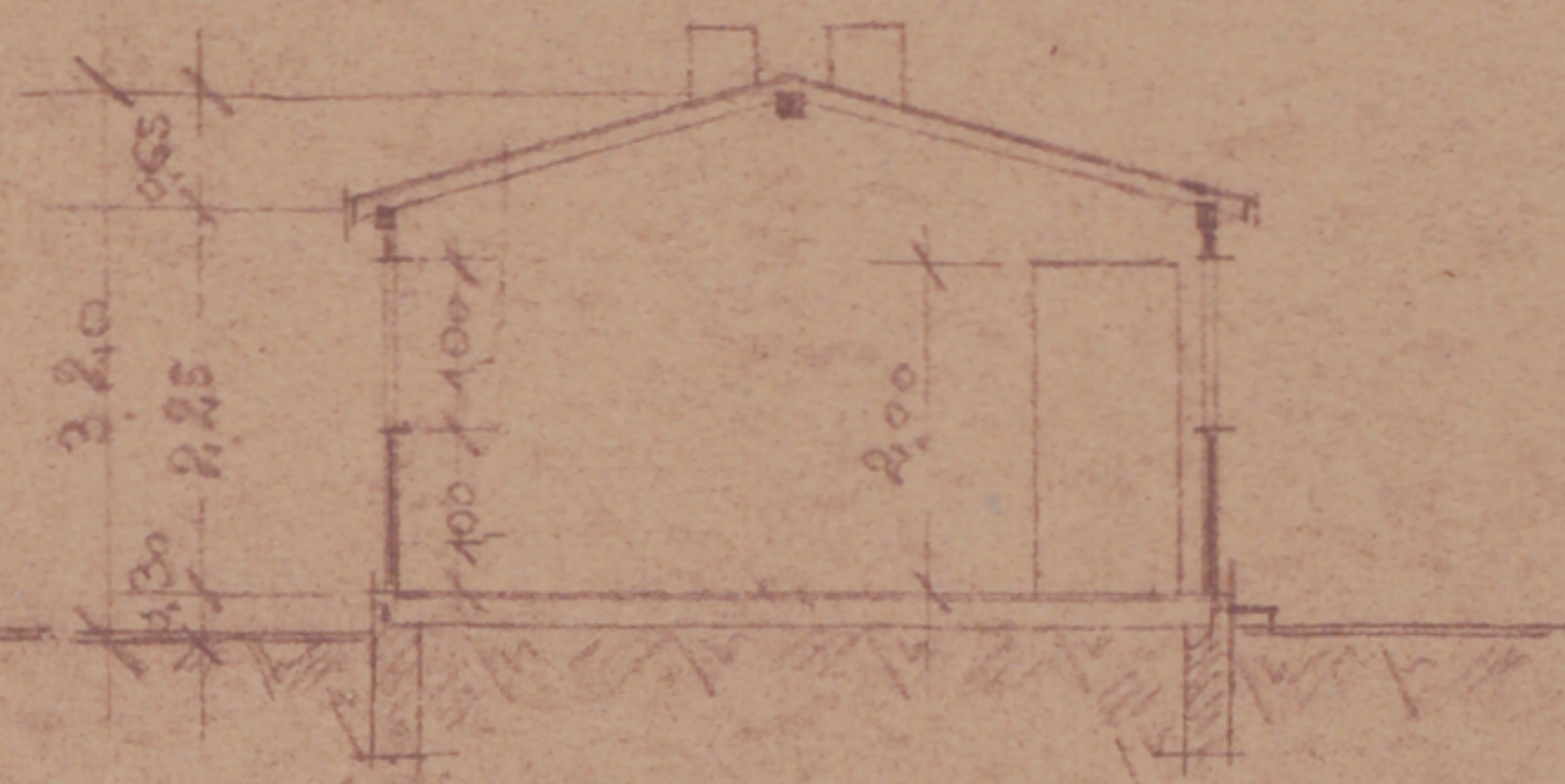
Schnitt a-b
