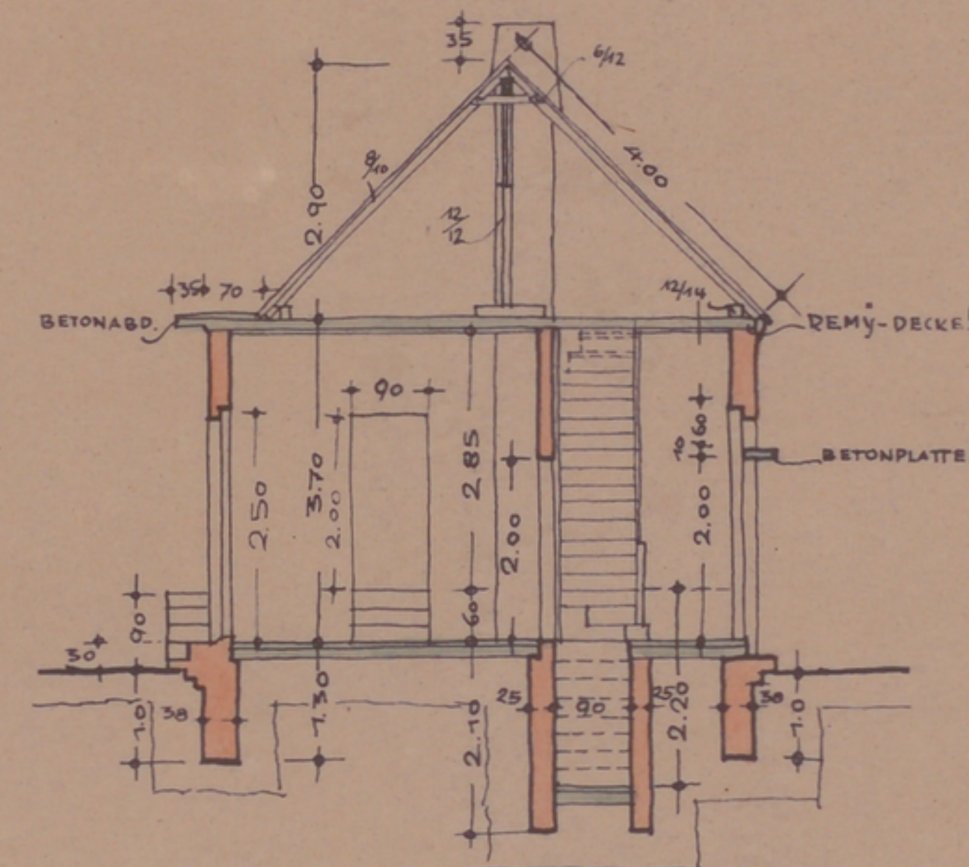
SCHNITT C-D
