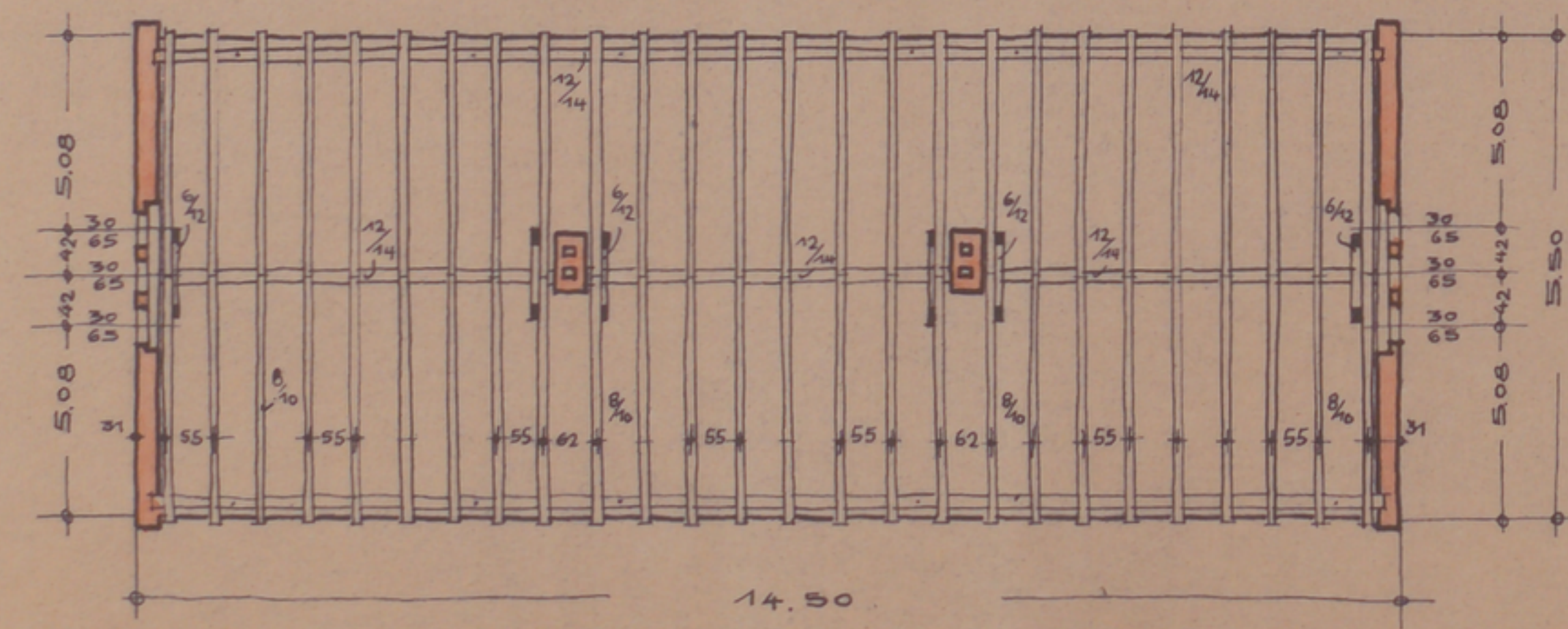
SPARRENLAGE.
