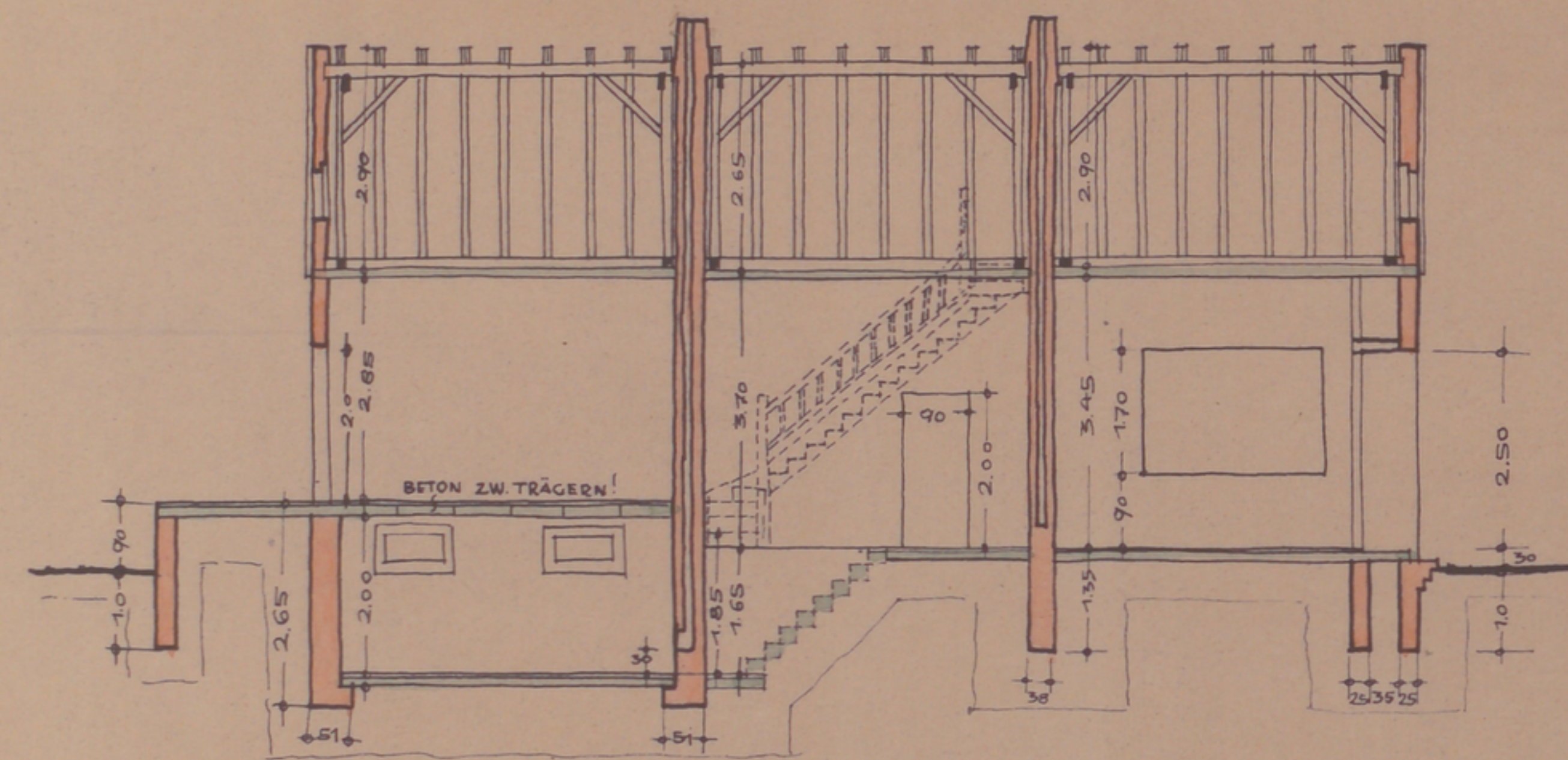
SCHNITT A-B.
